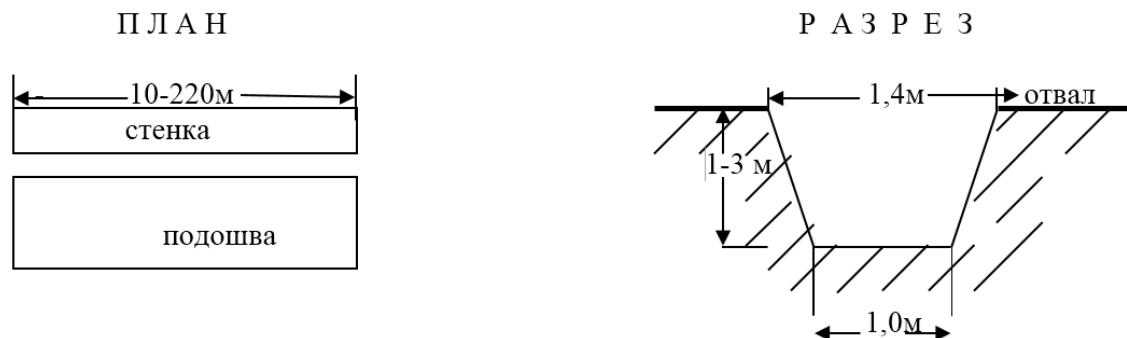
Рис. 9 Паспорт проходки канав глубиной до 2 м
