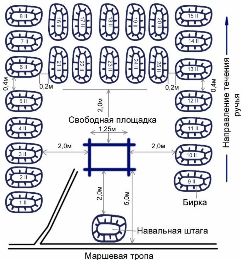
Рис. 7 – Схема выкладки и нумерации проходок
