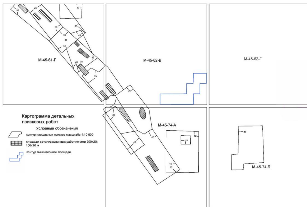
Рисунок 4 – Картограмма детальных поисковых работ
