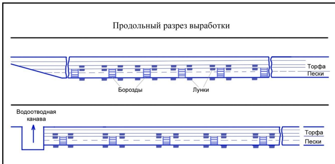
Рис. 8 План и продольный разрез проектируемой траншеи
