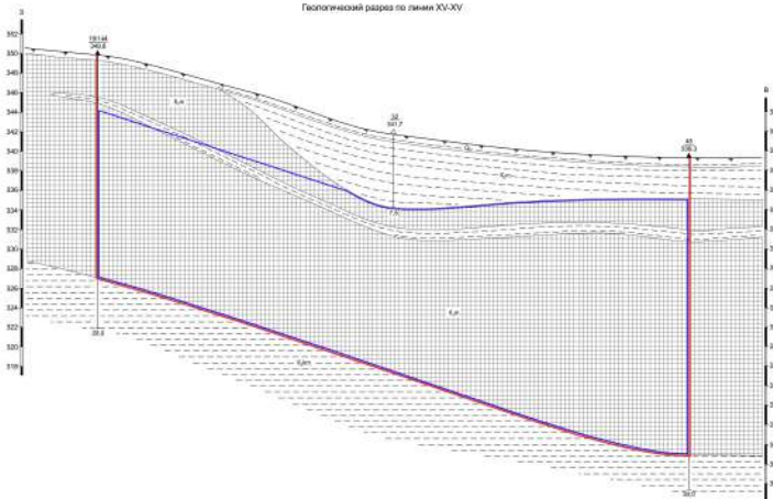
Геологический разрез по линии XV-XV
