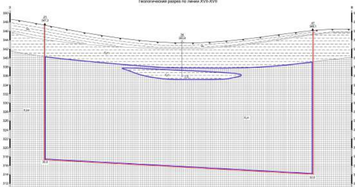
Геологический разрез по линии XVI-XVI
