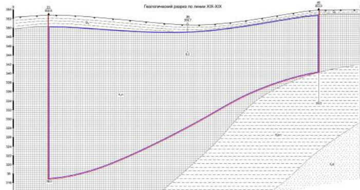
Геологический разрез по линии XIX-XIX
