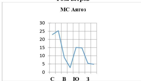
Роза ветров
