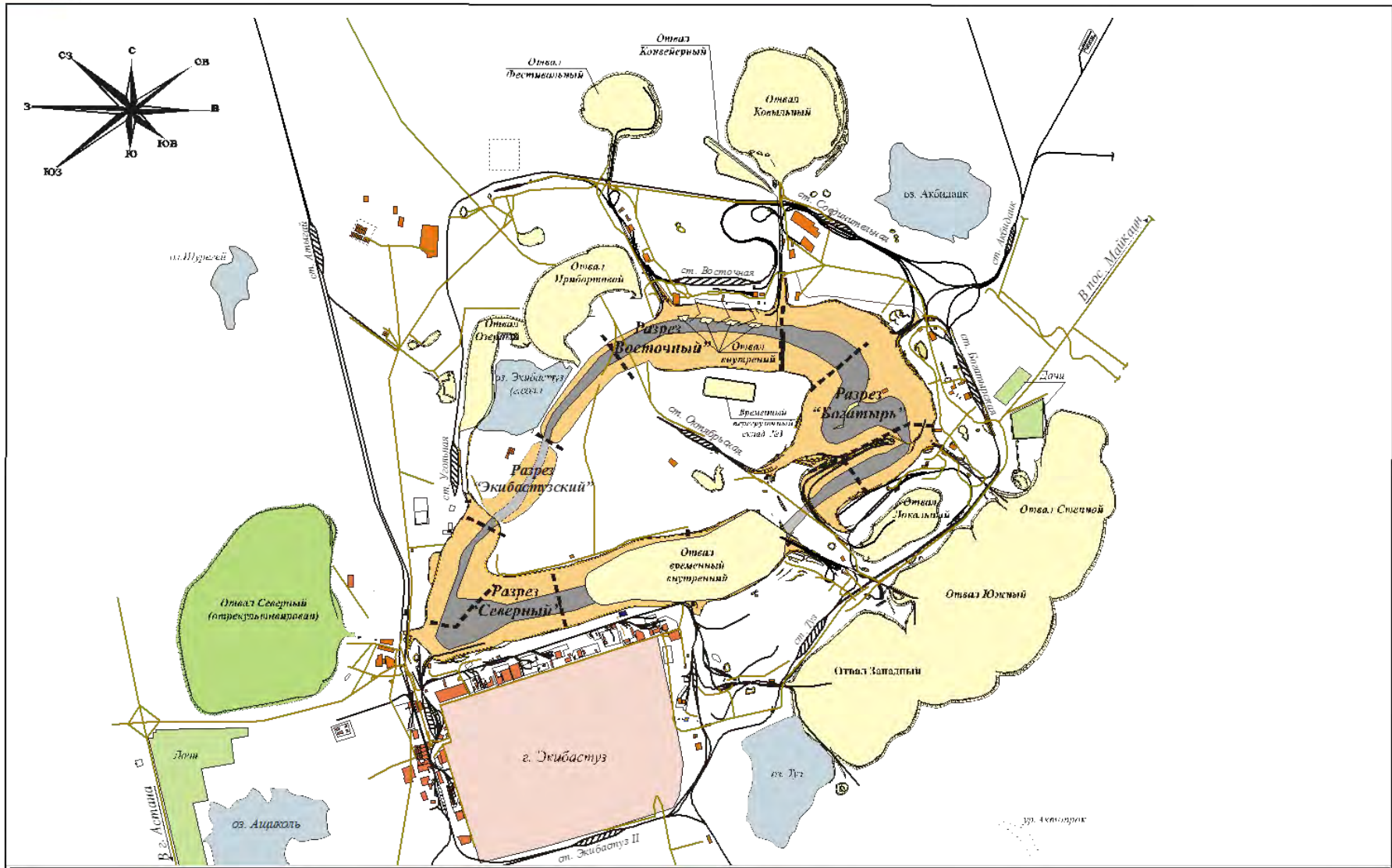
1.1-сурет Екібастұз көмір бассейнінің ахуалдық жоспары
