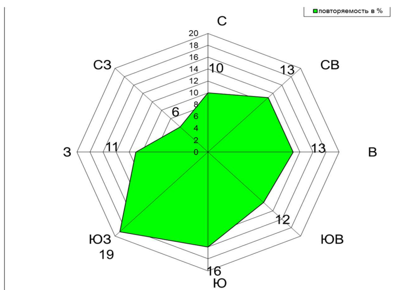
Рисунок 1.3 – Роза ветров
