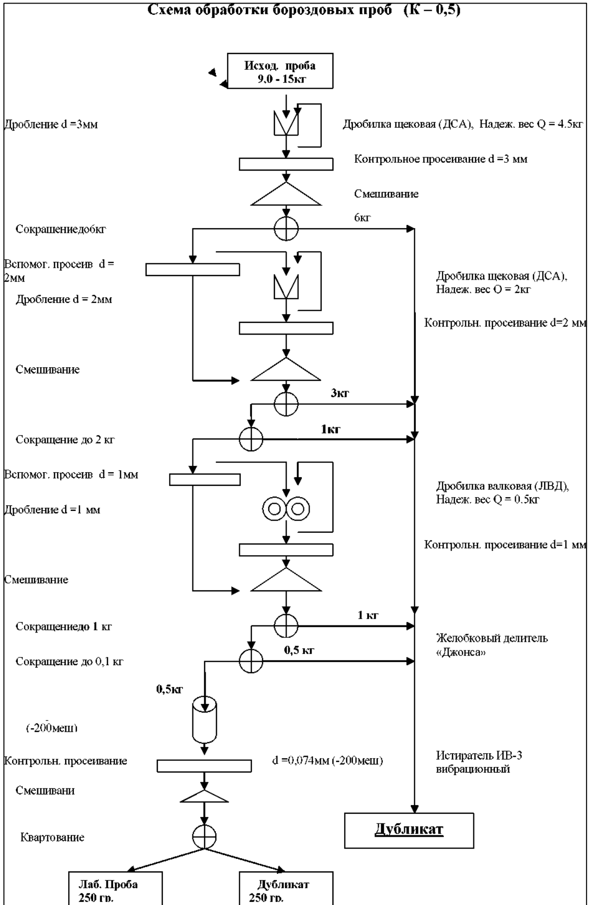
Рисунок 5.4.1 – Схема обработки бороздовых проб
