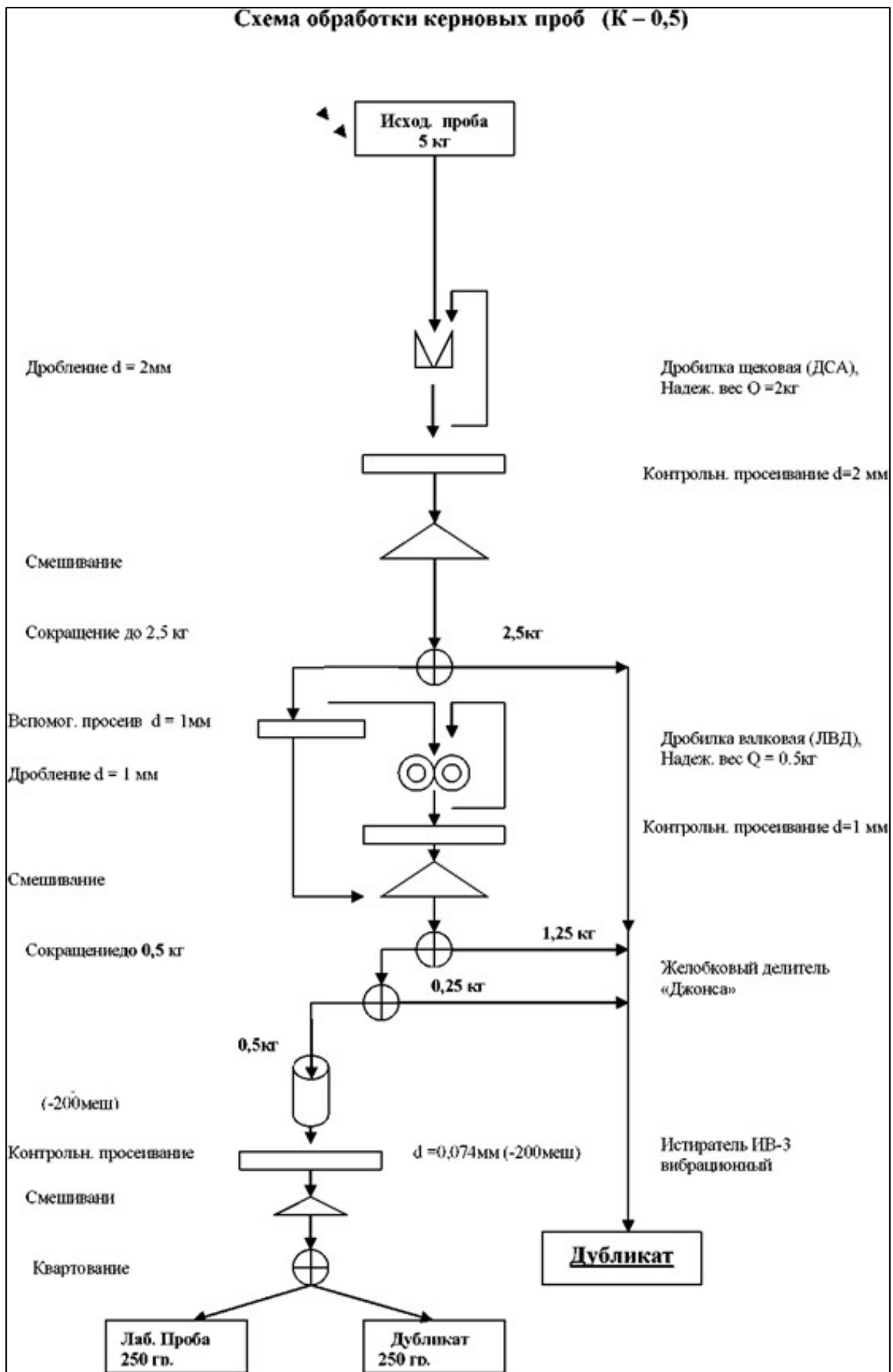
Рисунок 5.4.2 – Схема обработки керновых проб
