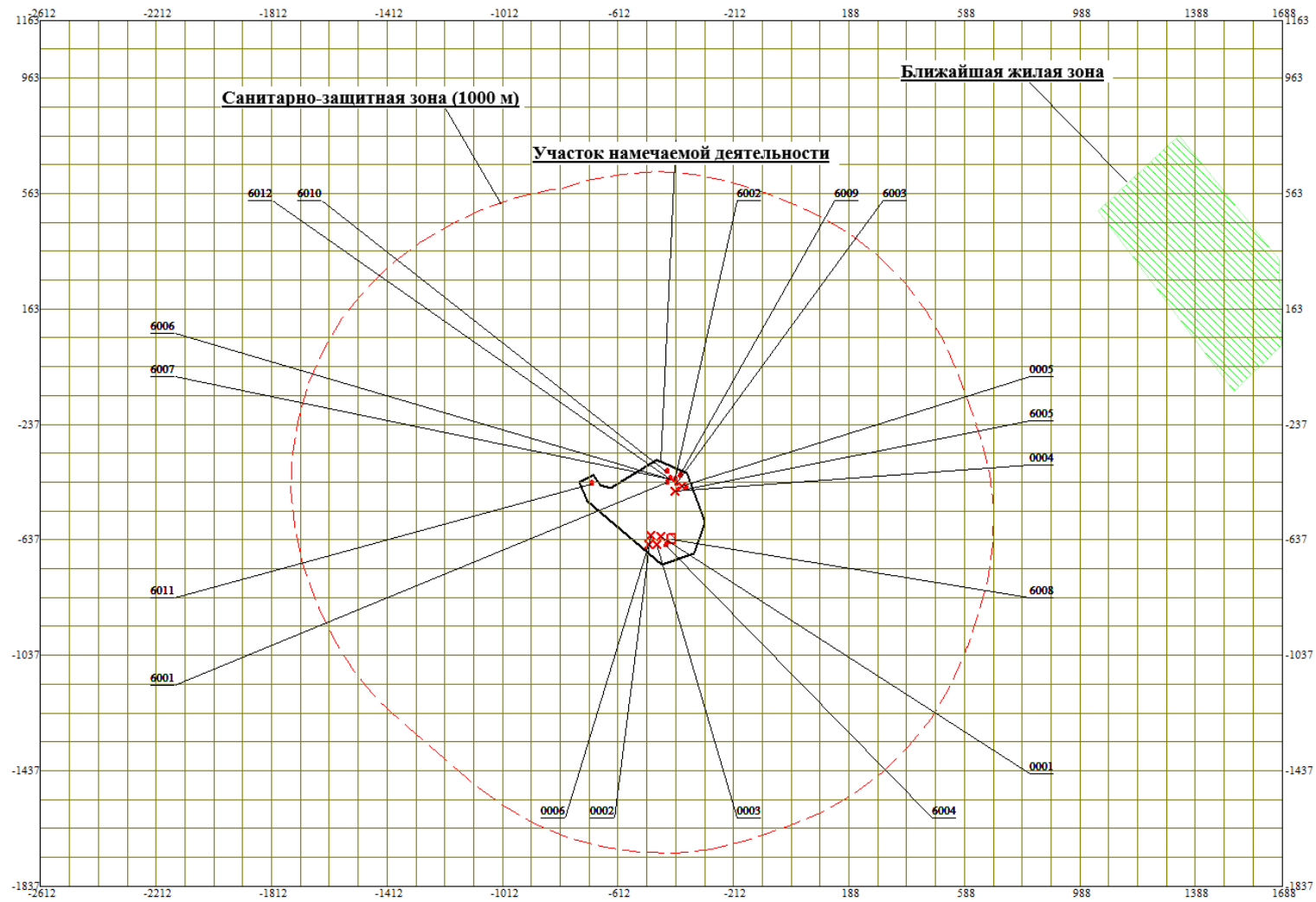
Рисунок 15.2 - Карта-схема участка проектирования с нанесенными источниками выбросов в атмосферу на период эксплуатации
