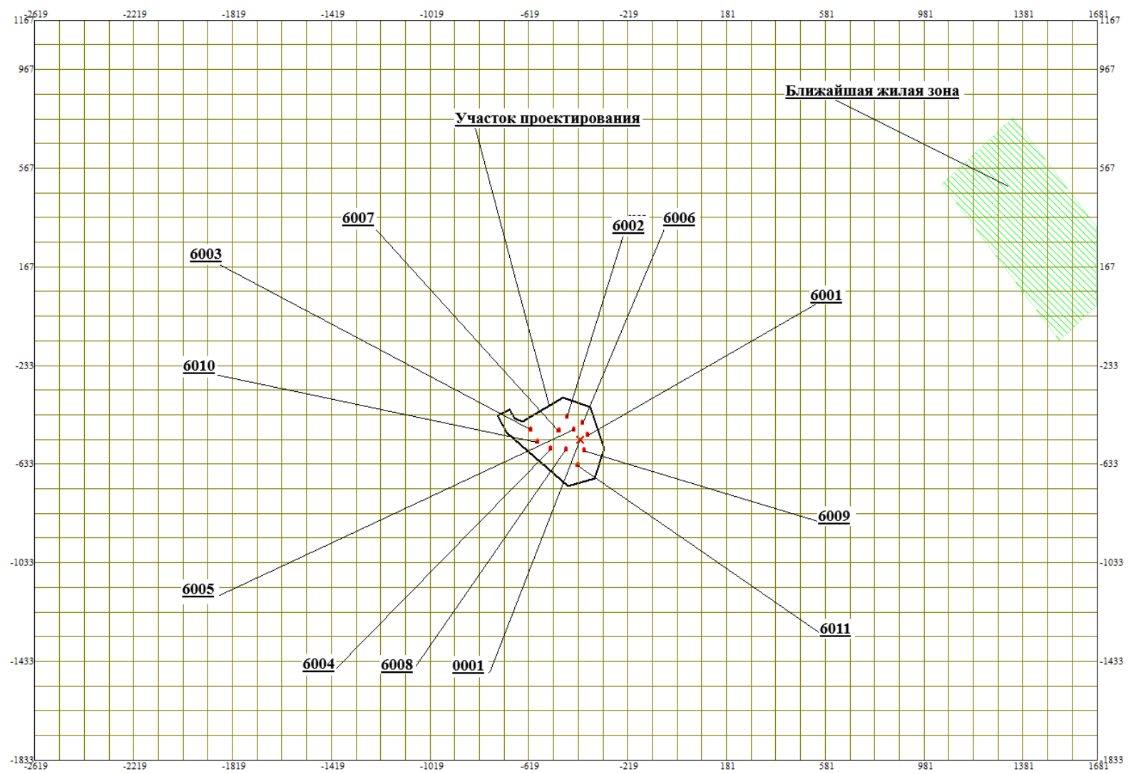
Рисунок 15.3 - Карта-схема участка проектирования с нанесенными источниками выбросов в атмосферу на период СМР
