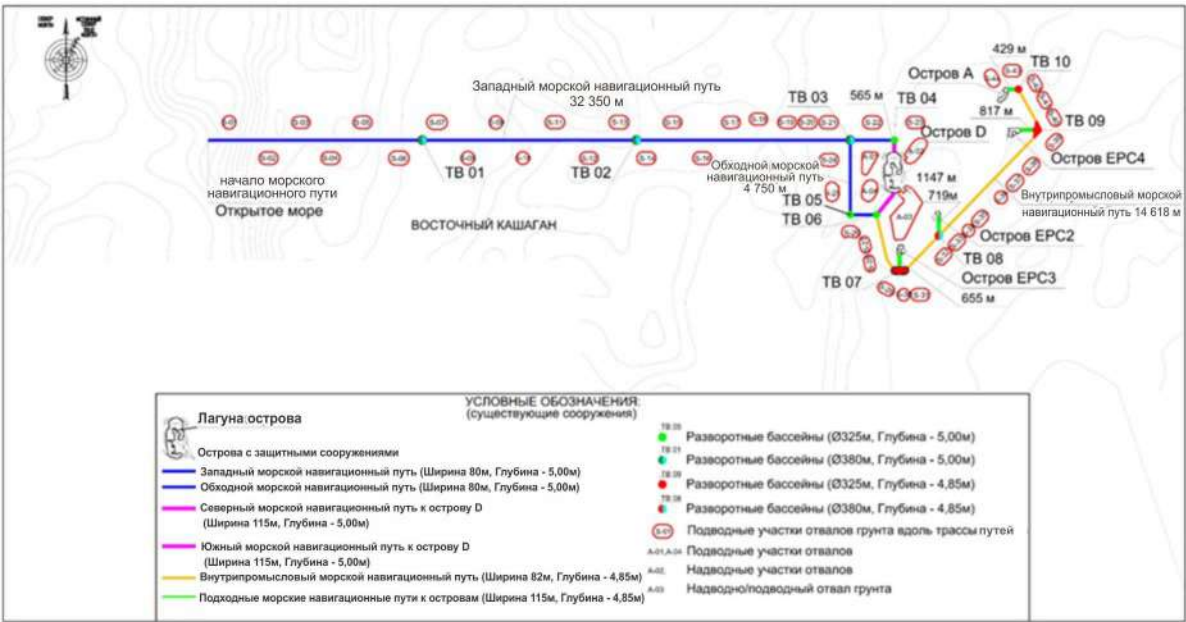
Рисунок 10.3 Схема существующих морских навигационных путей
