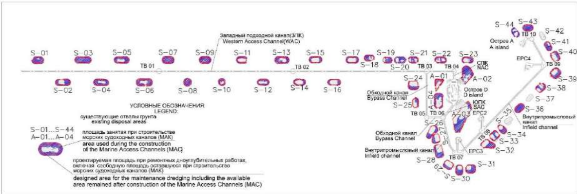
Рисунок 3.12 Площади существующих отвалов грунта
