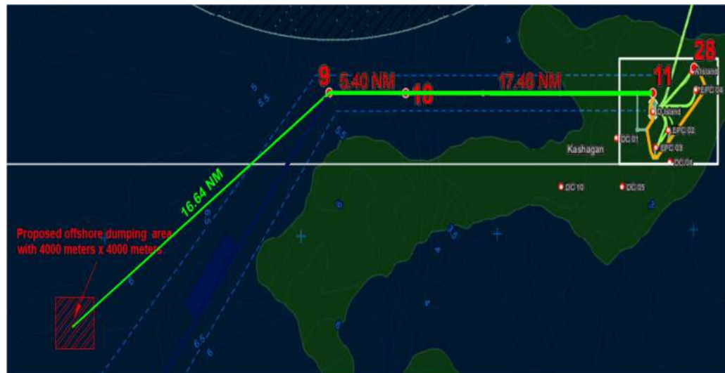
Рисунок 10.5 Схема транспортировки грунта в специально отведенную глубоководную зону Каспийского моря
