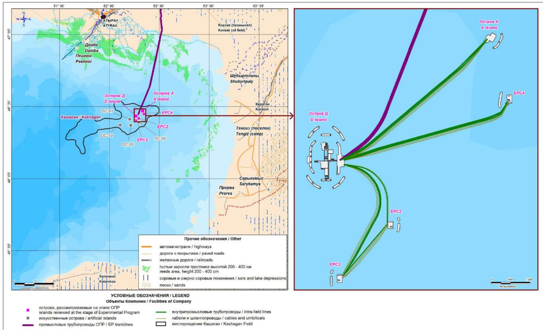
Рисунок 2.2.1 Ситуационная карта-схема района расположения Морского Комплекса
