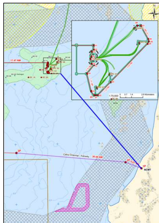
Рисунок 3.17 Маршрут СВП с порта Прорва до морских объектов
