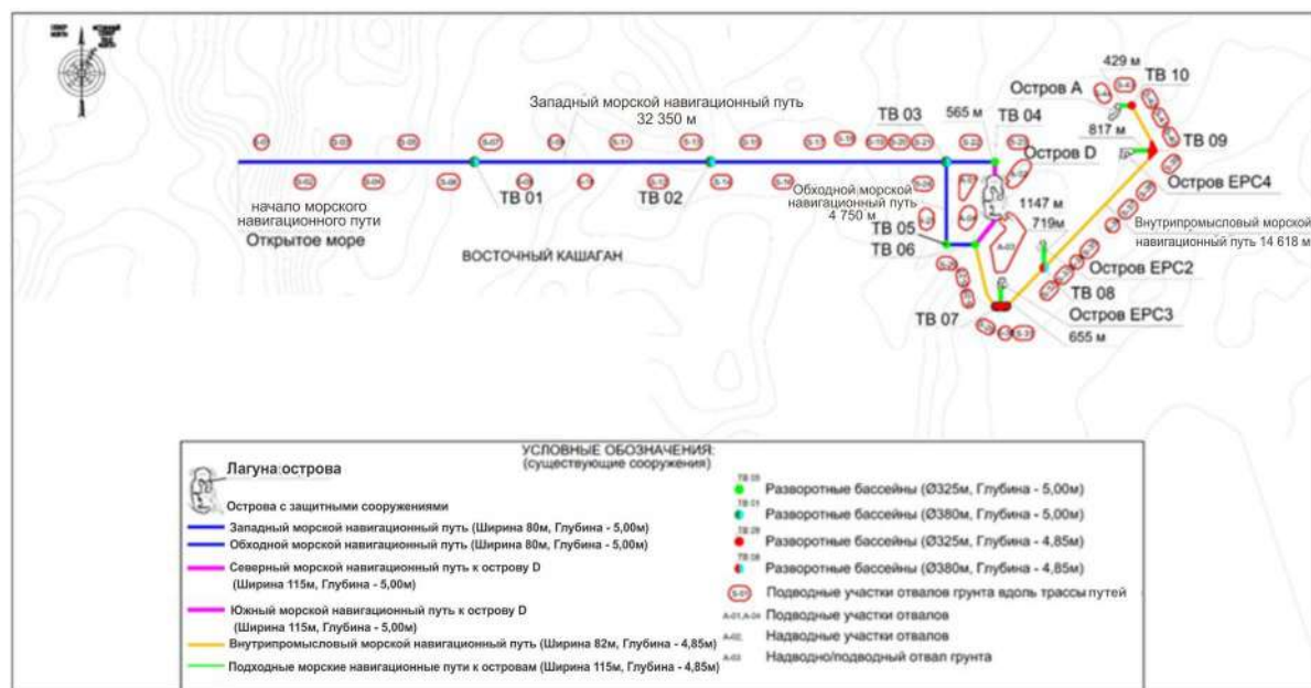
Рисунок 3.2 Схема существующих морских навигационных путей
