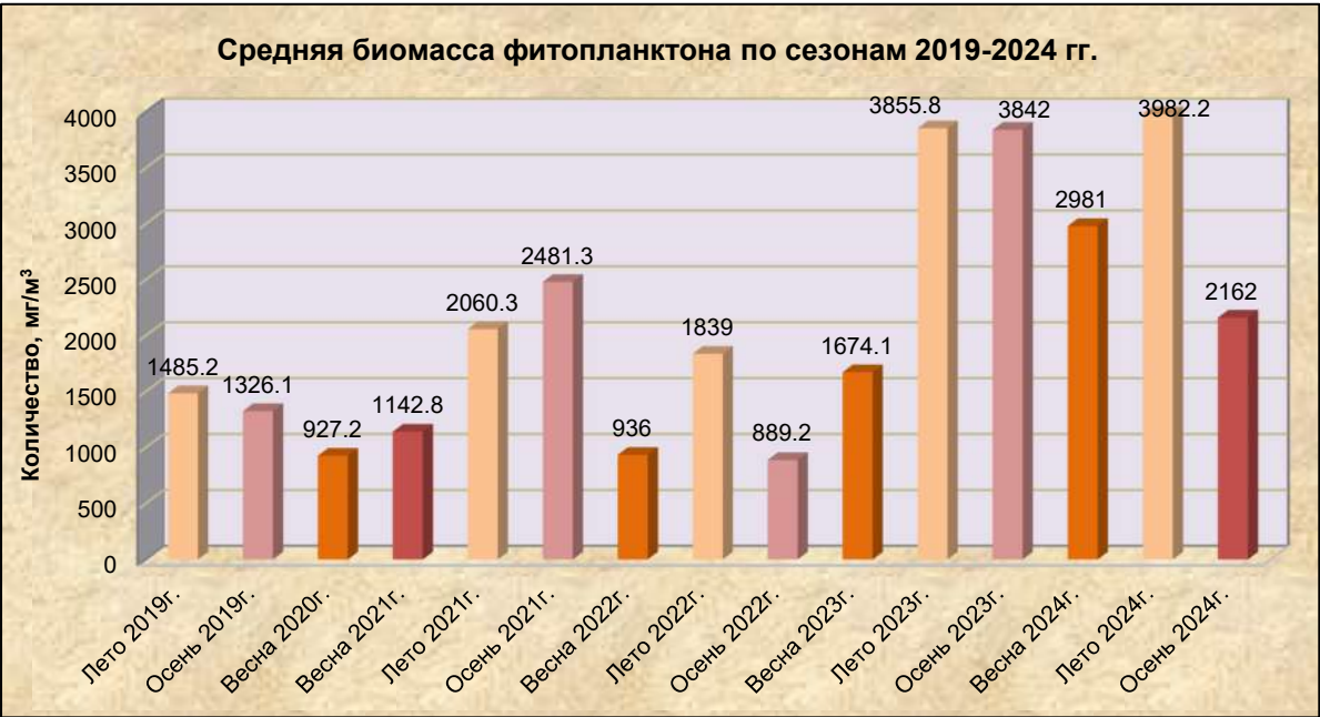
Рисунок 4.2.26 Биомасса фитопланктона на акватории морского навигационного пути в период исследований по сезонам в 2019-2024 гг.
