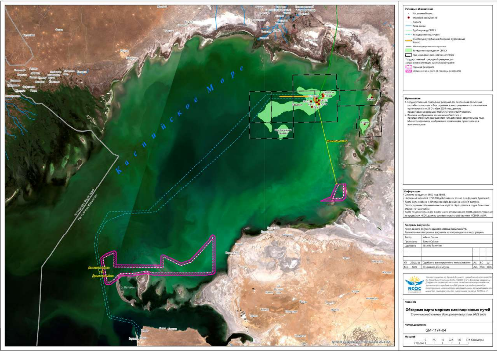
Рисунок 5.7.4 Государственный природный резерват (ГПР) «Каспий итбалыгы»
