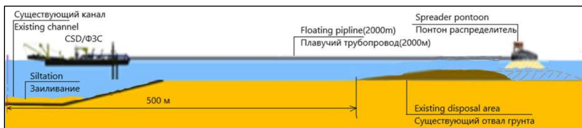
Рисунок 3.11 Концепция размещения извлеченного слоя заиливания земснарядом ФЗС в существующий подводный отвал
