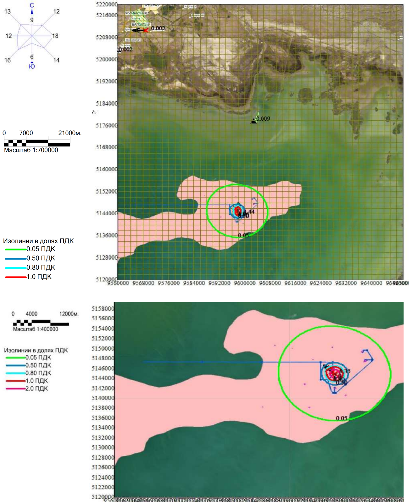
Рисунок 10.17 Изолинии приземных концентраций группы суммации азота и серы диоксида при проведении дноуглубления с использованием DOP при размещении грунта в существующих отвалах. Теплый период
