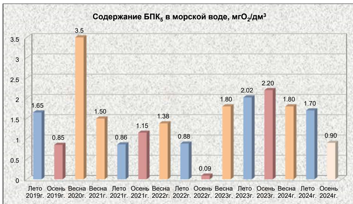
Рисунок 4.2.6 Средние содержания БПК 5 в воде акватории морского навигационного пути в 2019-2024 гг.
