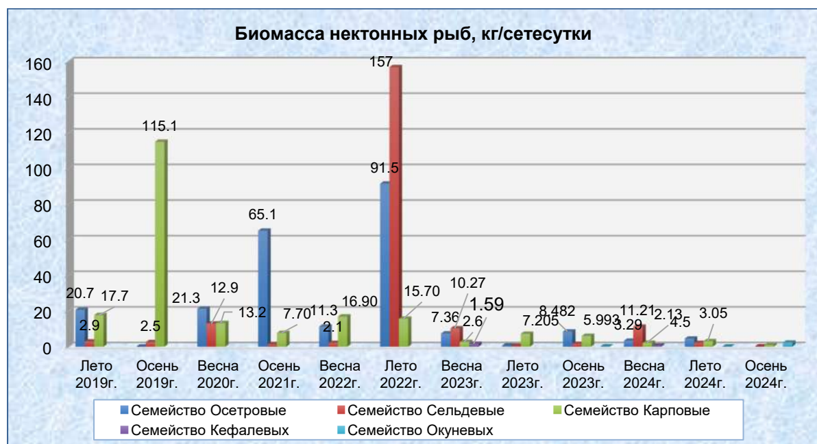
Рисунок 4.2.34 Распределение биомассы нектонных рыб по сезонам наблюдений на акватории морского навигационного пути в 2019-2024 гг.
