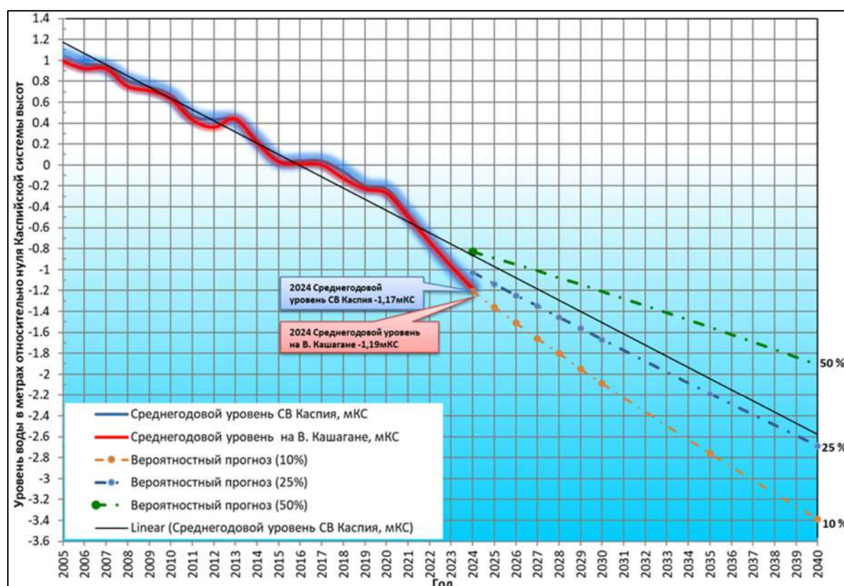
Рисунок 4.2.2 Среднегодовой уровень моря (2005-2024) Северо-Восточного Каспия и Восточного Кашагана
