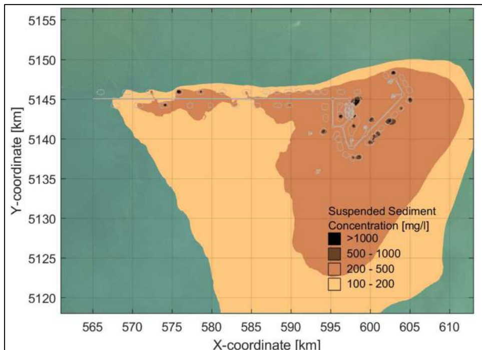
Рисунок 5.4.2 Результаты моделирования распространения шлейфа мутности в 2025 году
