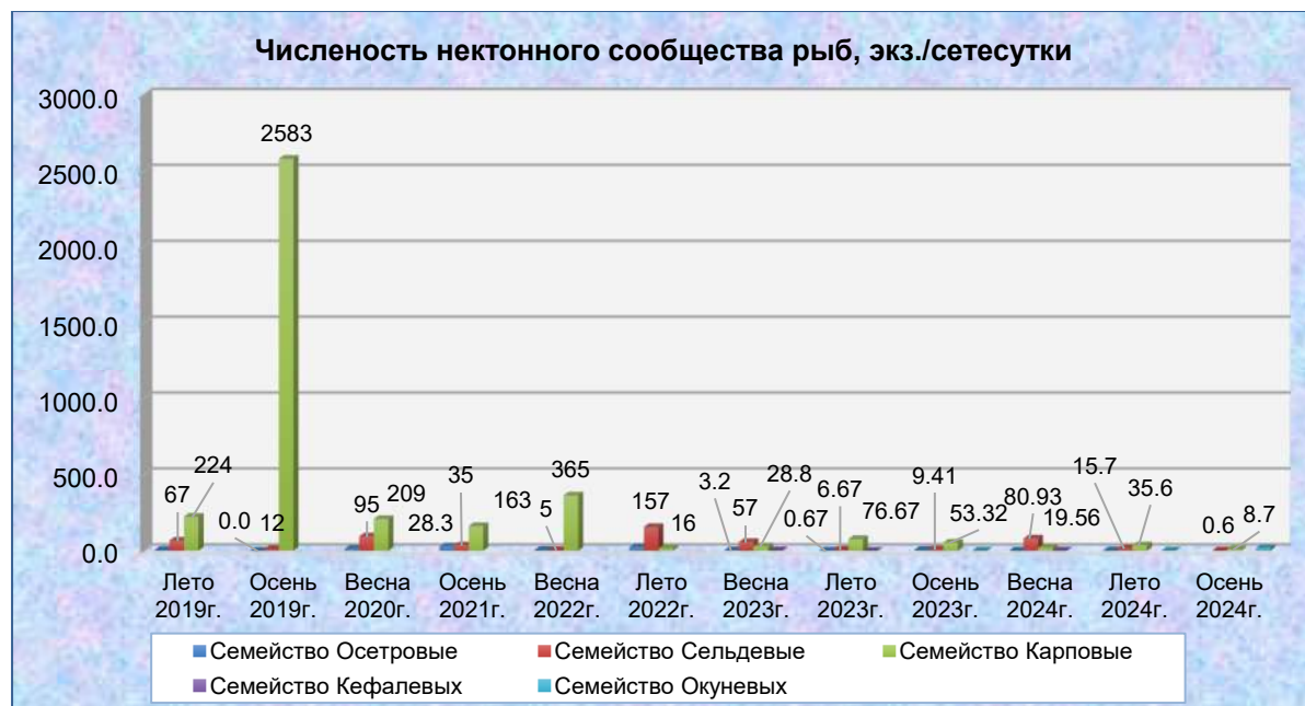
Рисунок 4.2.33 Распределение численности нектонных рыб по сезонам наблюдений на акватории морского навигационного пути в 2019-2024 гг.
