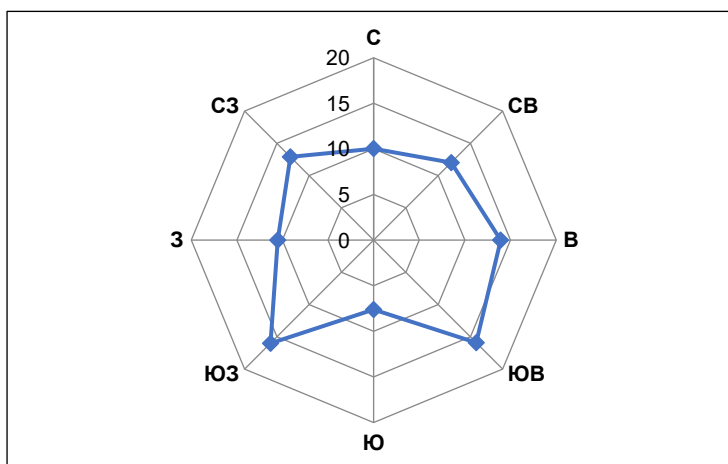
Рисунок 4.1.1 Роза ветров по м/с Пешной
