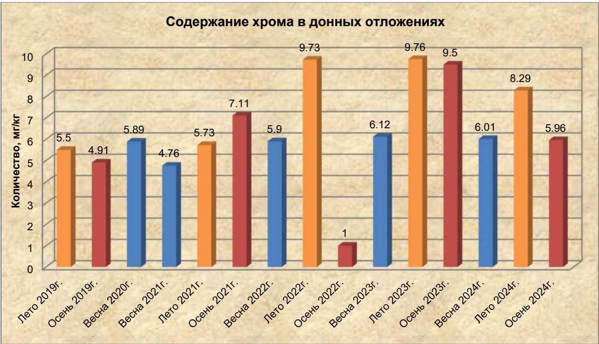
Рисунок 4.2.16 Средние содержания хрома в донных отложениях в районе морского навигационного пути по профилям KCR-1, KCR-2, KCR-3, KCR-4, KCR-7 по сезонам в 2019-2024 гг.
