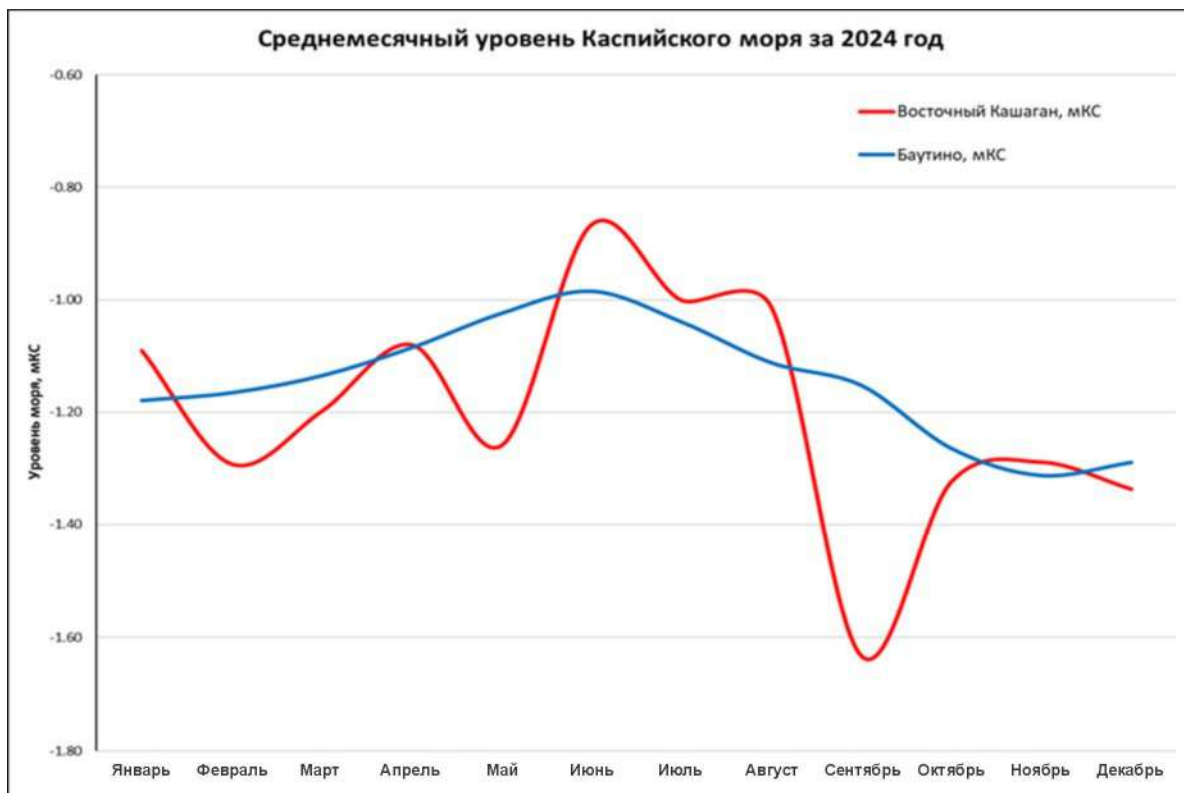
Рисунок 4.2.3 Среднемесячные значения уровня моря на участках Кашаган и Баутино
