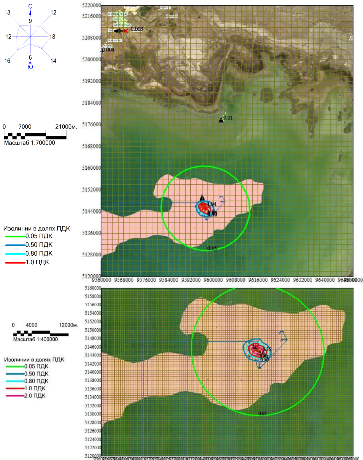
Рисунок 10.18 Изолинии приземных концентраций группы суммации азота и серы диоксида при проведении дноуглубления с использованием DOP, шаланды и позиционной баржи при транспортировке извлеченного грунта на глубину или на берег. Теплый период
