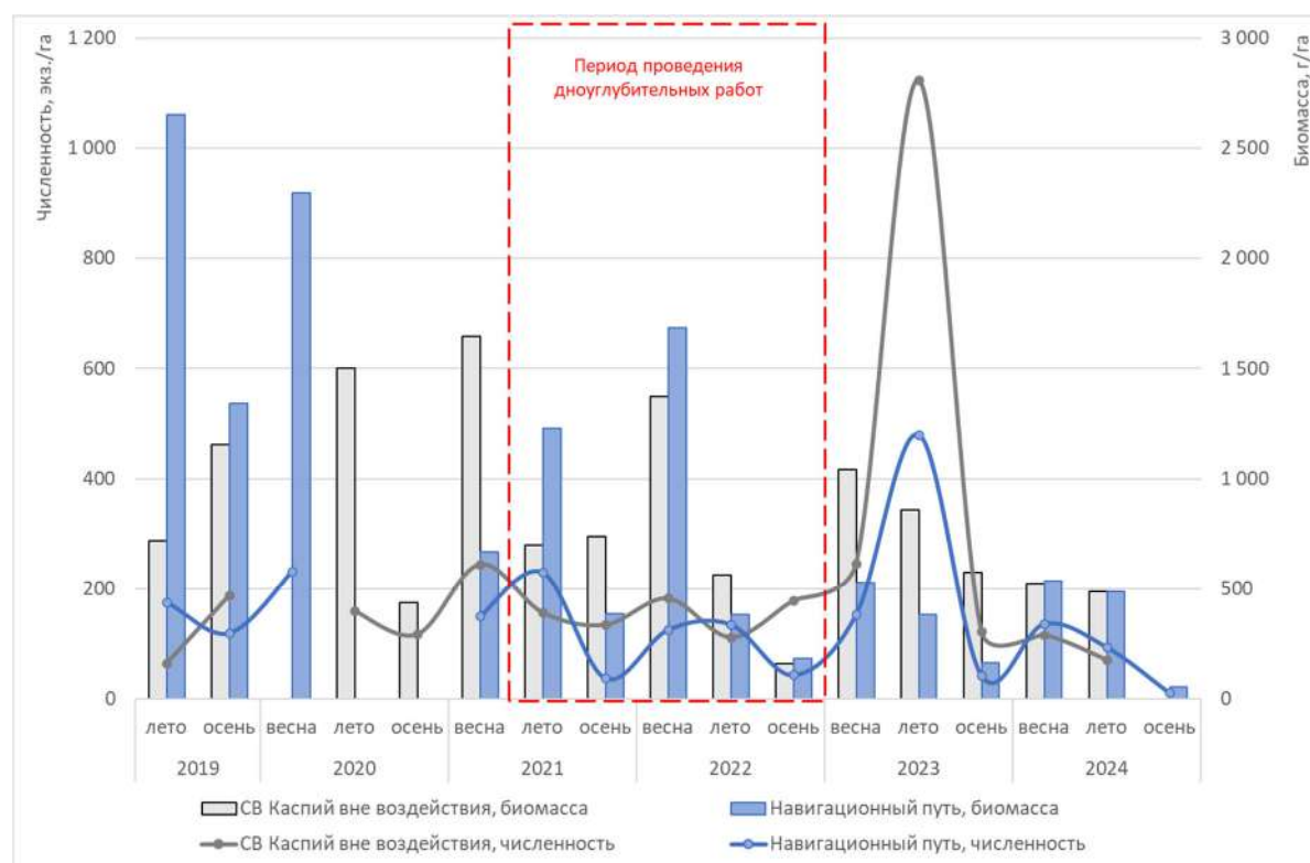
Рисунок 5.9.8 Динамика количественных показателей бенто-пелагического сообщества рыб во время исследований в районе проведения дноуглубительных работ
