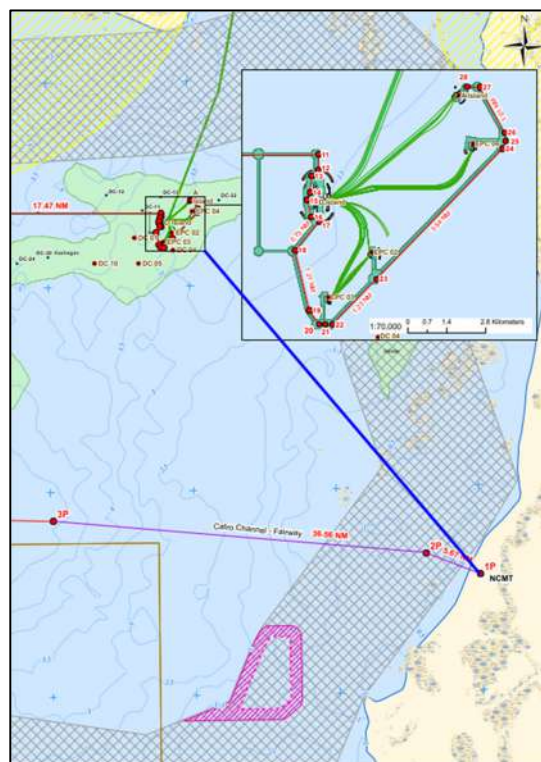
Рисунок 10.16 Маршрут СВП с порта Прорва до морских объектов
