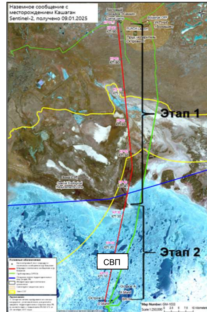
Рисунок 10.15 Карта поэтапного строительства Наземного Соединения
