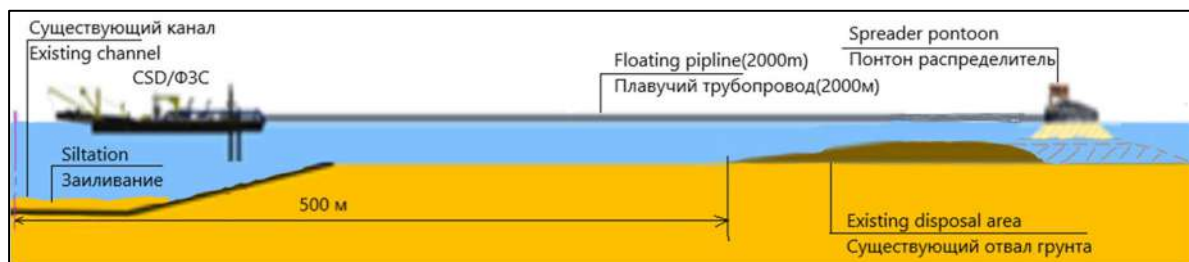
Рисунок 10.12 Концепция размещения извлеченного слоя заиливания земснарядом ФЗС в существующий подводный отвал
