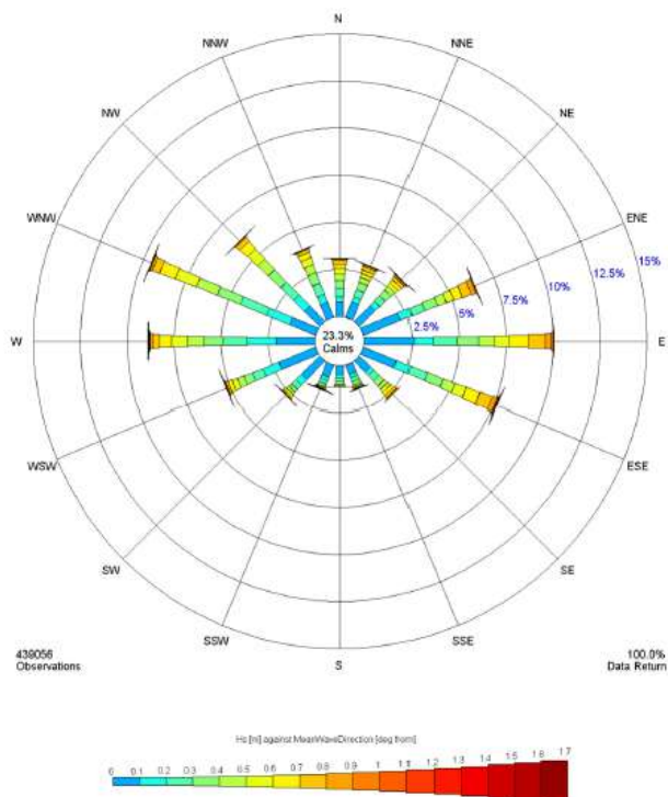
Рисунок 4.2.4 Диаграмма для определения высоты волны ( H_s ) и среднего направление волны 4
