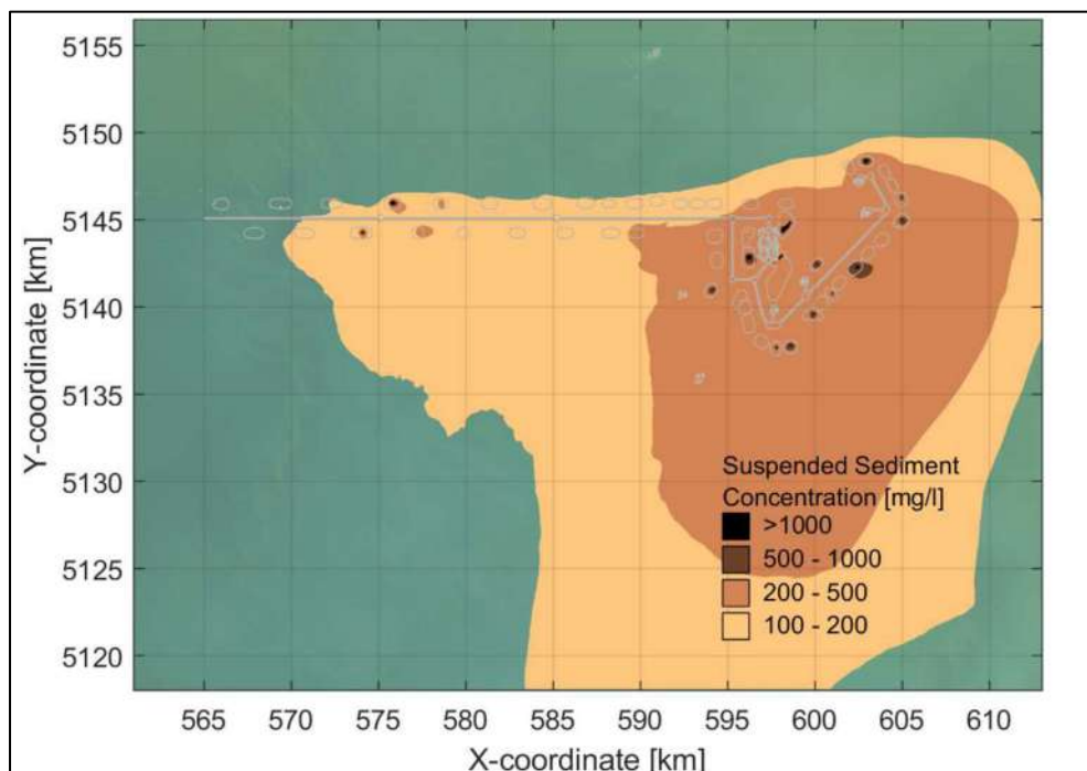
Рисунок 5.4.3 Результаты моделирования распространения шлейфа мутности в 2026 году
