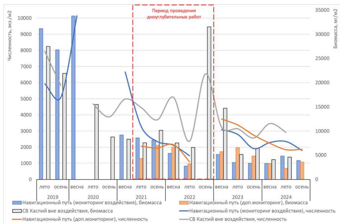
Рисунок 5.9.4 Динамика количественных показателей макрозообентоса во время исследований в районе проведения дноуглубительных работ
