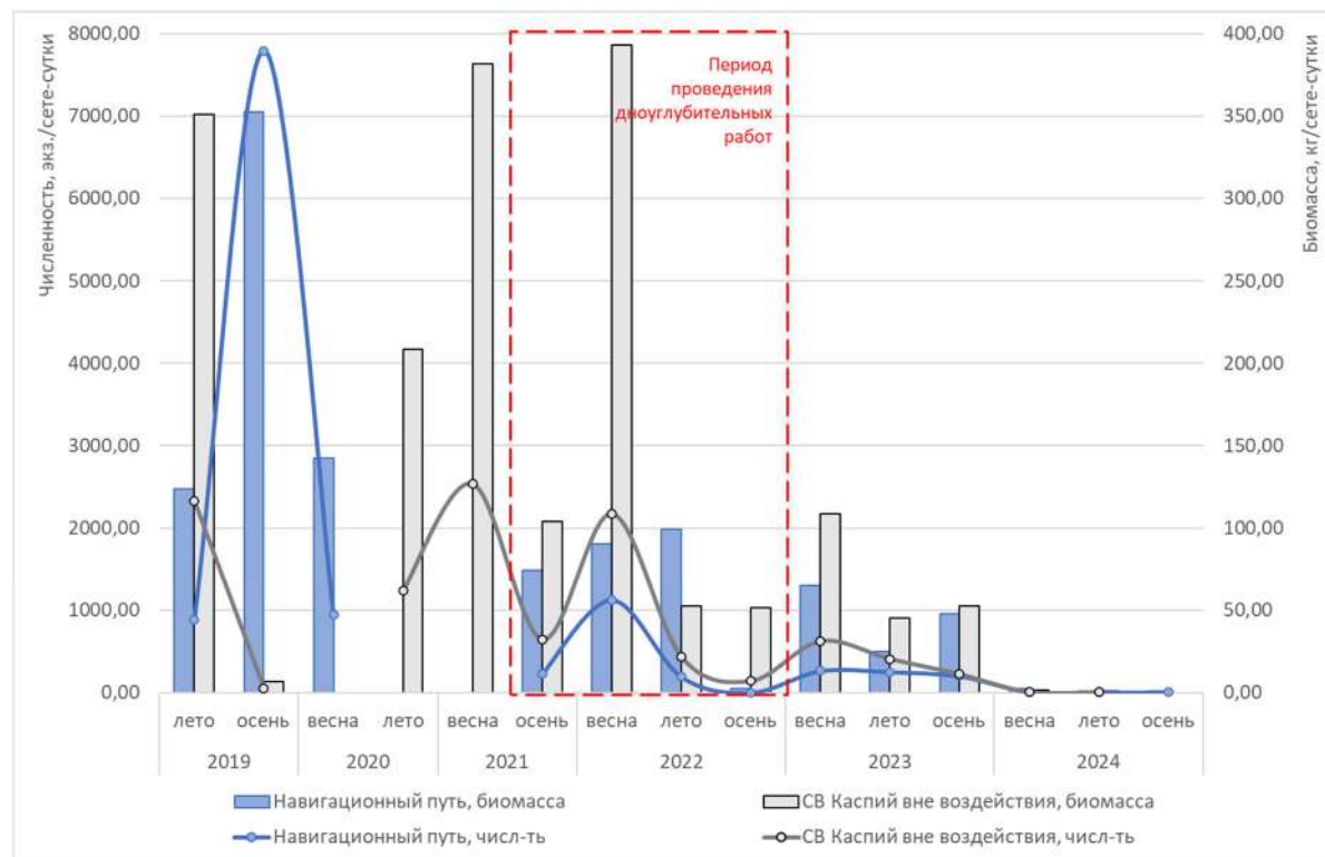
Рисунок 5.9.9 Динамика количественных показателей нектонного сообщества рыб во время исследований в районе проведения дноуглубительных работ
