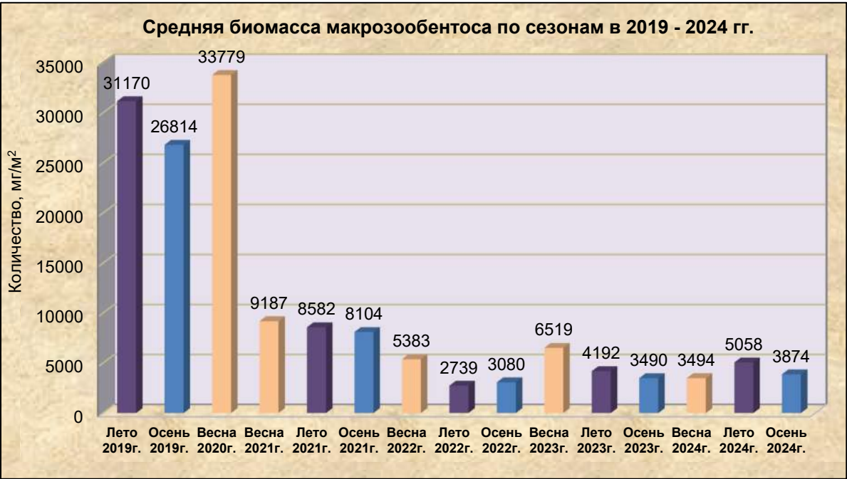
Рисунок 4.2.32 Биомасса макрозообентоса на акватории морского навигационного пути в период исследований по сезонам в 2019-2024 гг.
