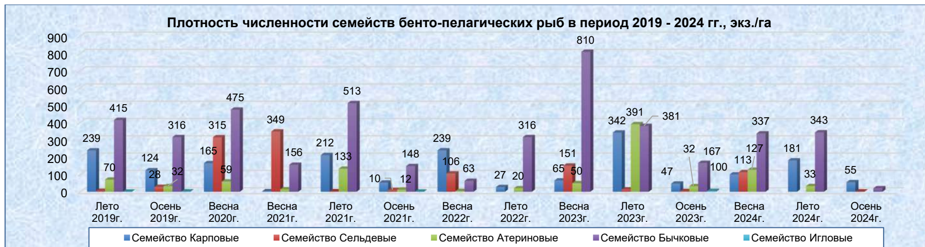
Рисунок 4.2.35 Распределение численности бенто-пелагических рыб по сезонам наблюдений на акватории морского навигационного пути в 2019–2024 гг.
