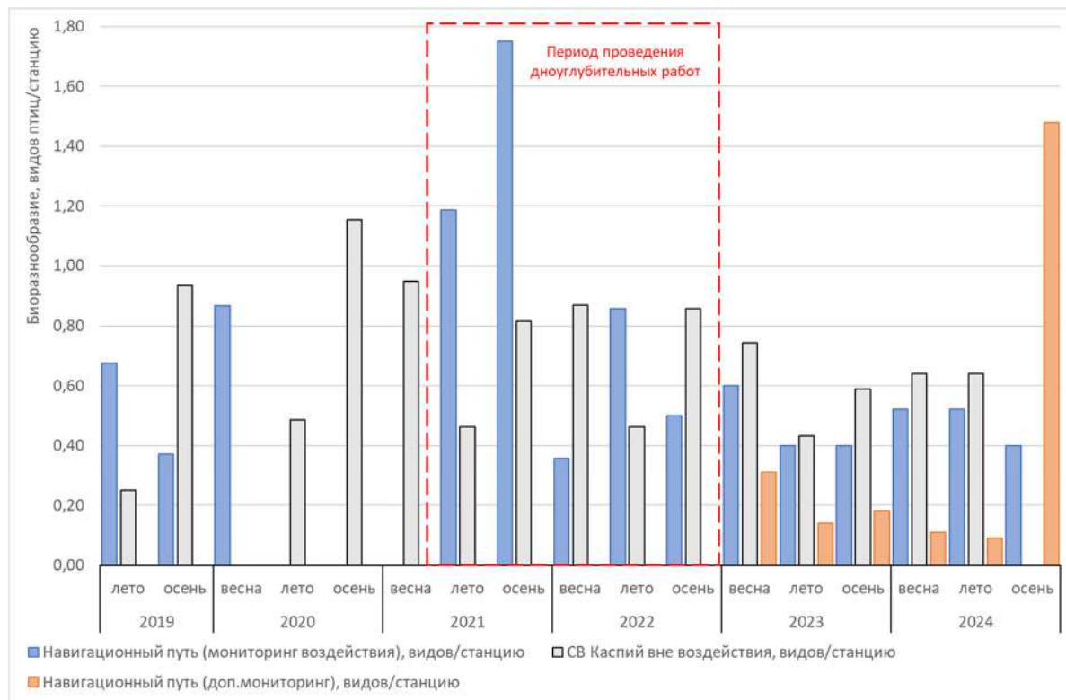
Рисунок 5.9.7 Биоразнообразие птиц во время исследований в районе проведения дноуглубительных работ
