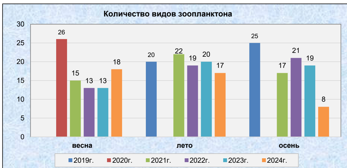
Рисунок 4.2.27 Количество видов зоопланктона, обнаруженных в период экологических исследований в 2019-2024 гг. на акватории морского навигационного пути
