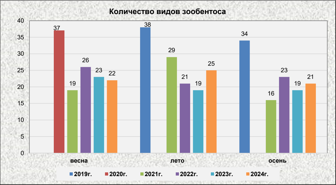
Рисунок 4.2.30 Количество видов зообентоса, обнаруженных в период исследований в 2019-2024 гг. на акватории морского навигационного пути
