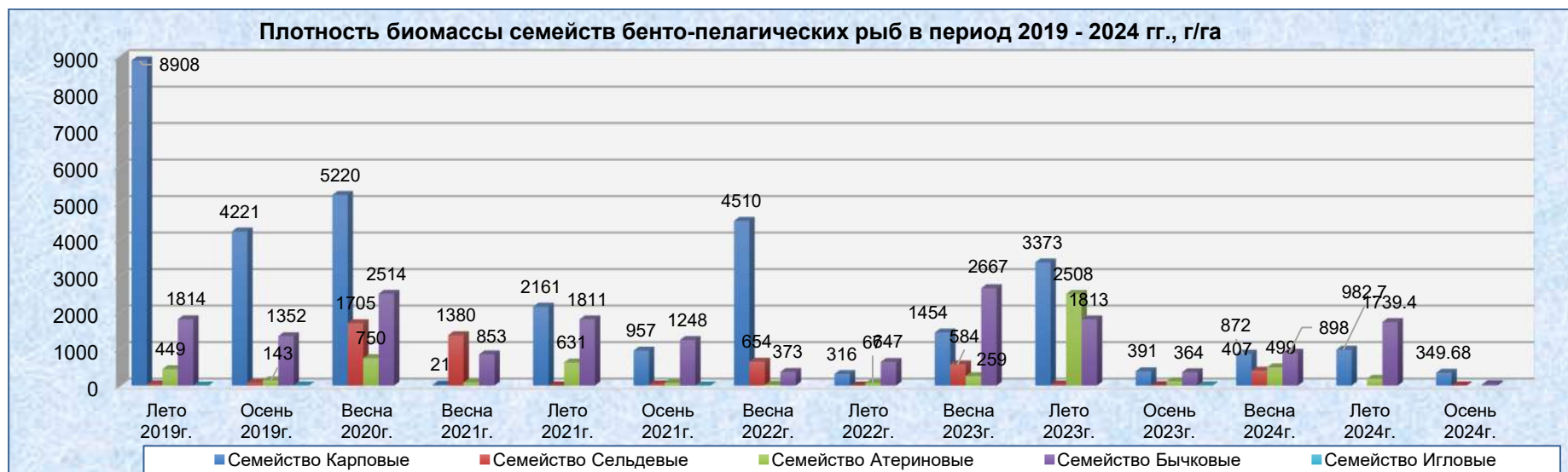
Рисунок 4.2.36 Распределение биомассы бенто-пелагических рыб по сезонам наблюдений на акватории морского навигационного пути в 2019–2024 гг.
