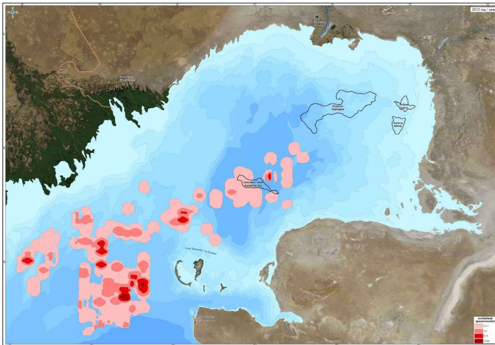
Рисунок 5.7.5 Зона экологической чувствительности обитания тюленей для рождения и щенных лежбищ тюленей
