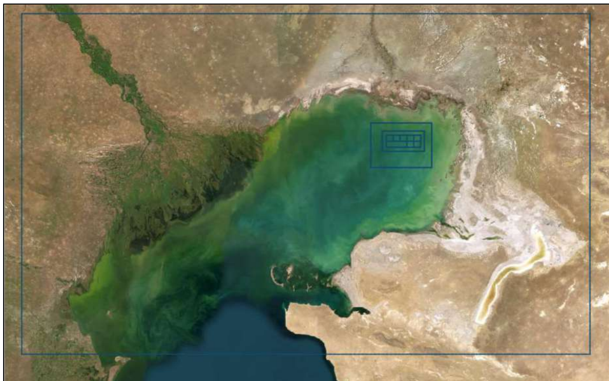
Рисунок 5.4.1 Расширение модельных доменов
