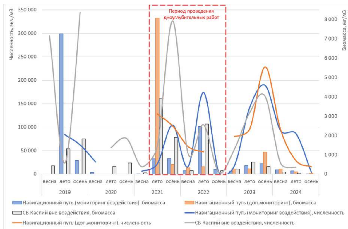
Рисунок 5.9.3 Динамика количественных показателей зоопланктона во время исследований в районе проведения дноуглубительных работ
