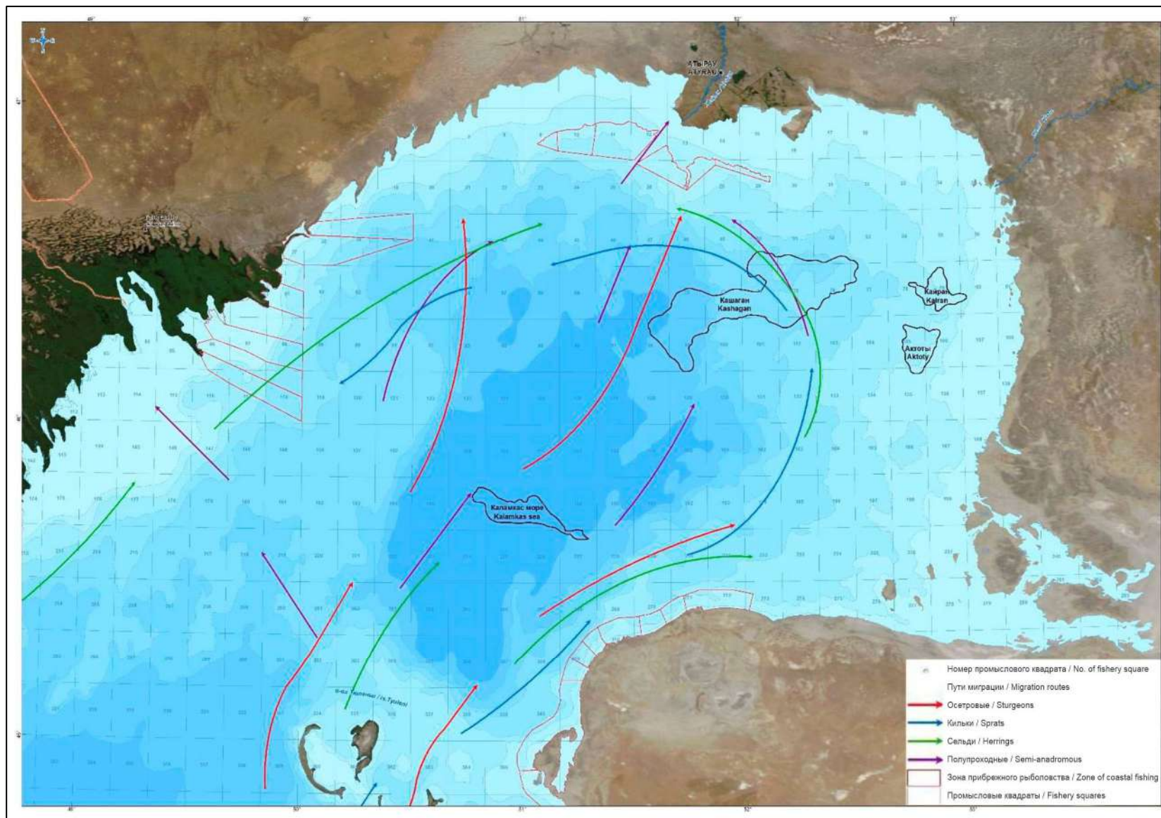
Рисунок 5.7.2 Пути миграции рыб
