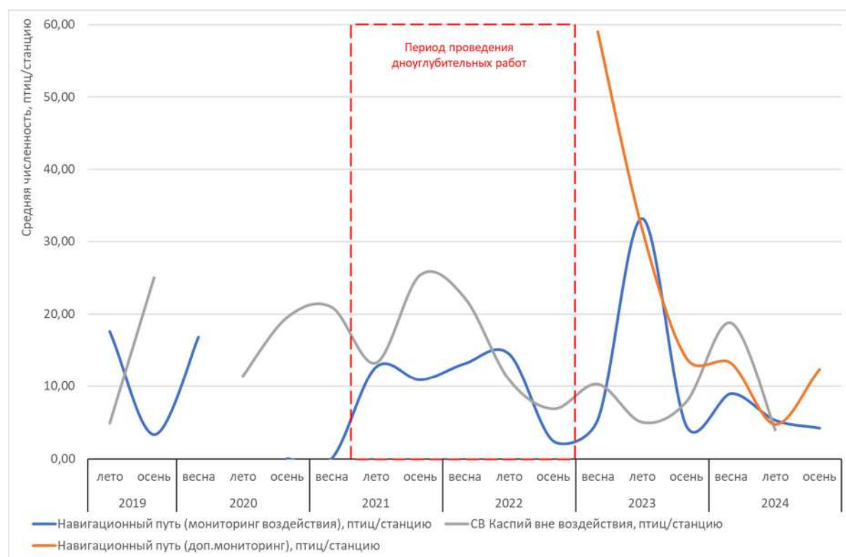
Рисунок 5.9.6 Численность птиц во время исследований в районе проведения дноуглубительных работ
