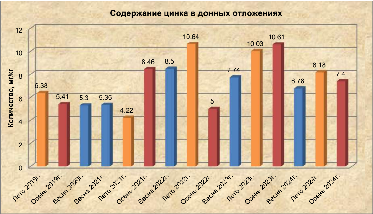
Рисунок 4.2.22 Средние содержания цинка в донных отложениях в районе морского навигационного пути по профилям KCR-1, KCR-2, KCR-3, KCR-4, KCR-7 по сезонам в 2019-2024 гг.
