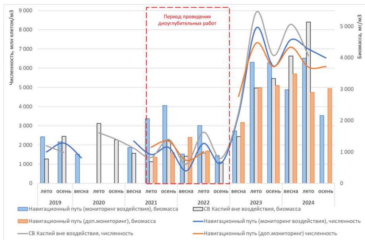
Рисунок 5.9.2 Динамика количественных показателей фитопланктона во время исследований в районе проведения дноуглубительных работ
