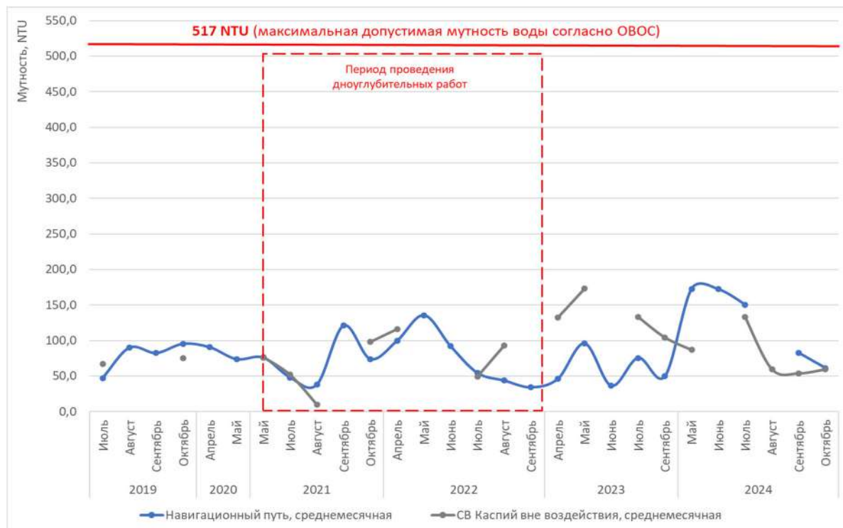
Рисунок 5.9.1 Колебания среднемесячной мутности воды во время исследований в районе проведения дноуглубительных работ
