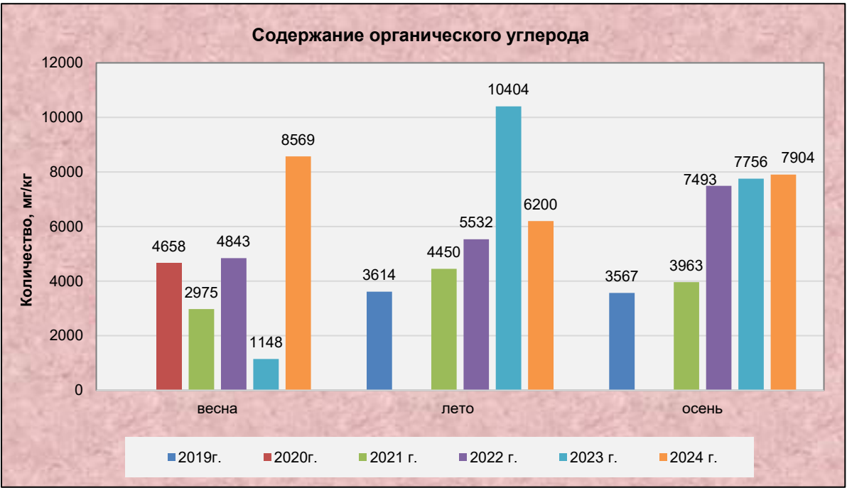
Рисунок 4.2.11 Среднее содержание органического углерода в донных отложениях в районе морского навигационного пути в период 2019–2024 гг.
