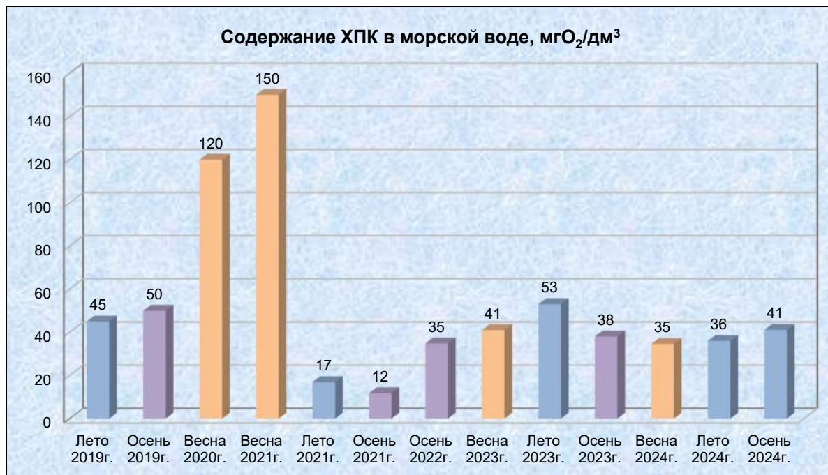
Рисунок 4.2.7 Средние содержания ХПК в воде акватории участка в 2019-2024 гг.
