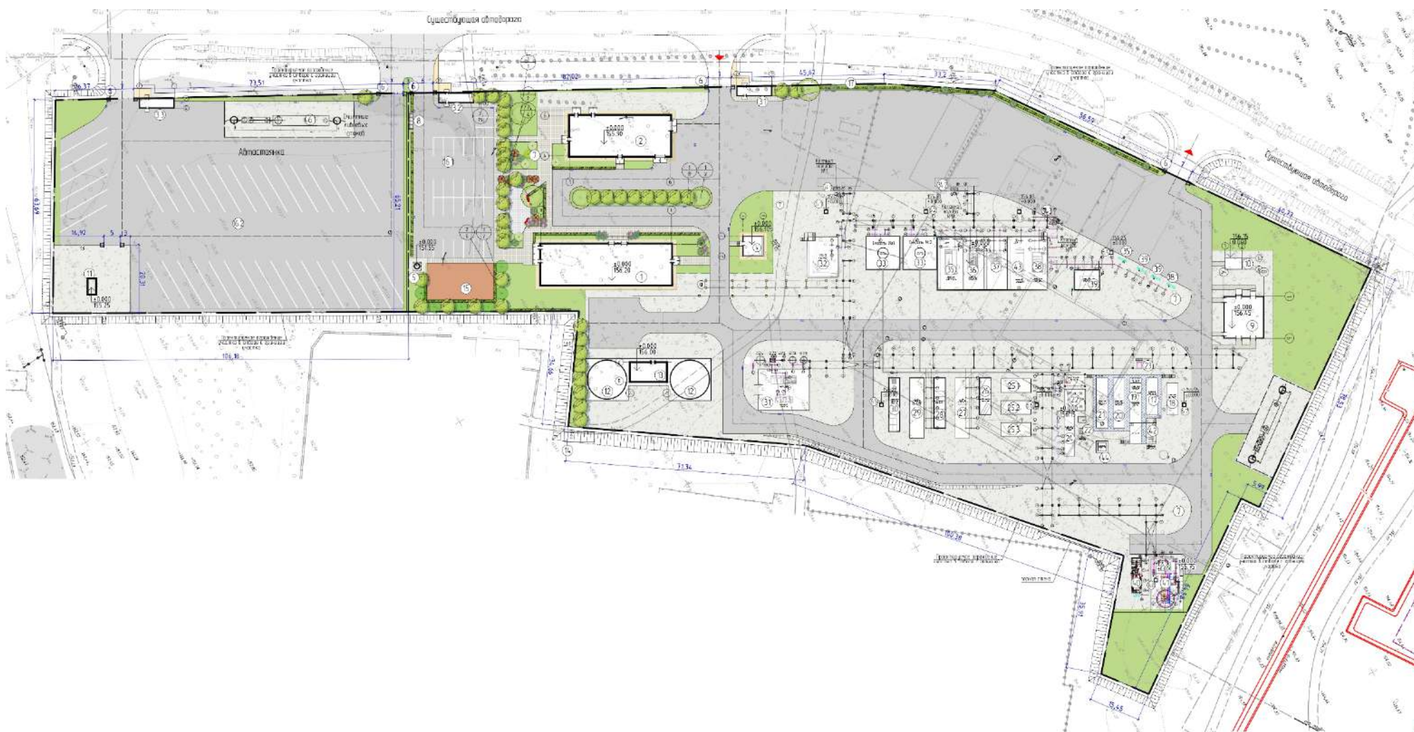
Рис. 6 План благоустройства
