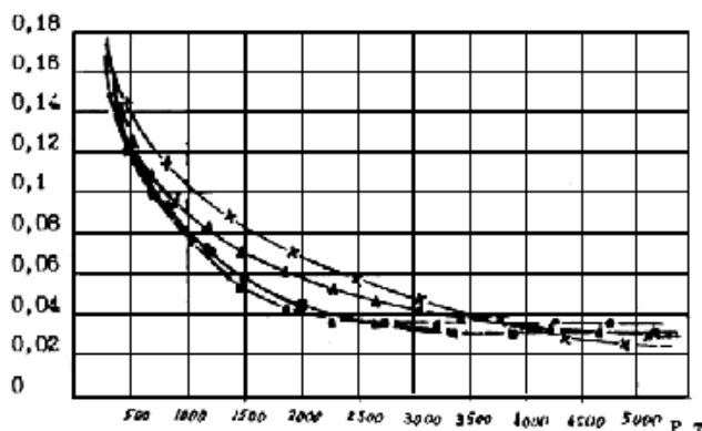
Рисунок 16.3 – Изменение значений удельных выбросов СО грузовыми тепловозами в зависимости от весов перевозимых поездов
