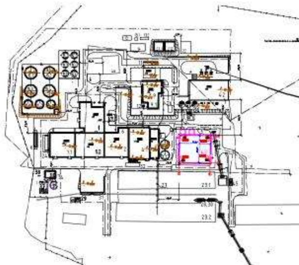
Рисунок 1 – Генеральный план
