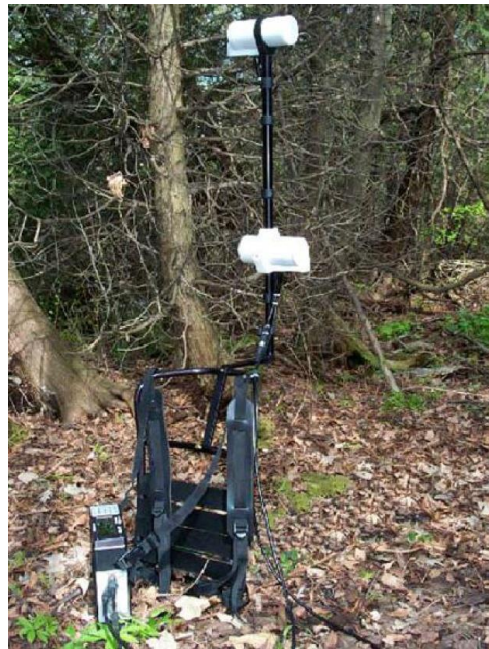
Рис. 5.11.1 Магнитометр GSM-19 в рабочем положении
