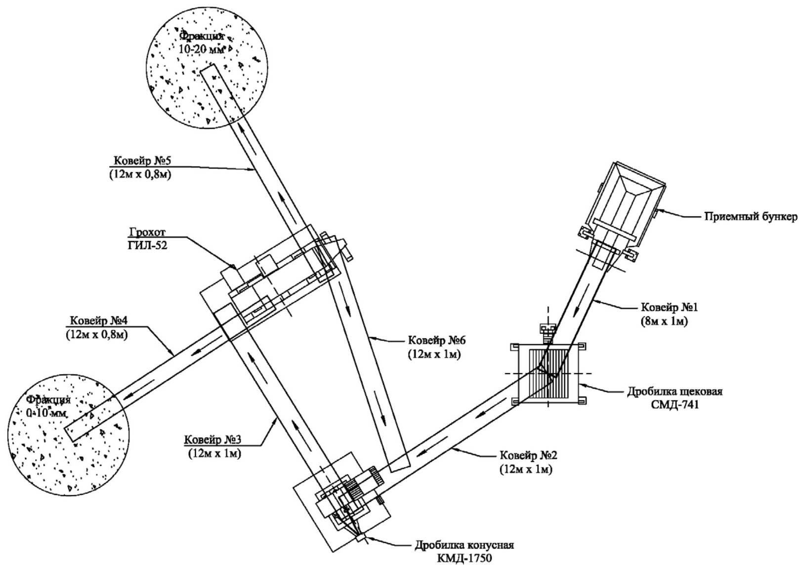
Рис. 2.6 Технологическая схема ДСК
