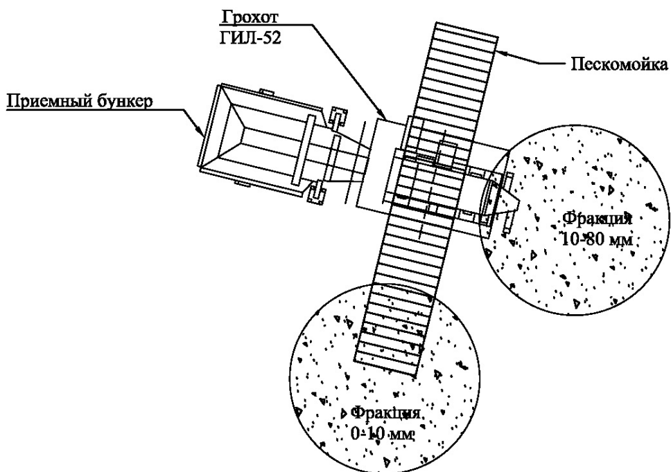
Рис. 2.5 Технологическая схема ПК №2
