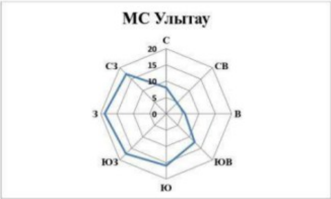
Повторяемость направлений ветра и штилей, %
