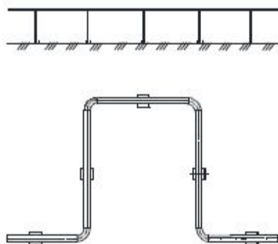
Рисунок 3.5 – Компенсатор
