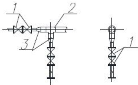
Рисунок 3.4 - Узел соединения
