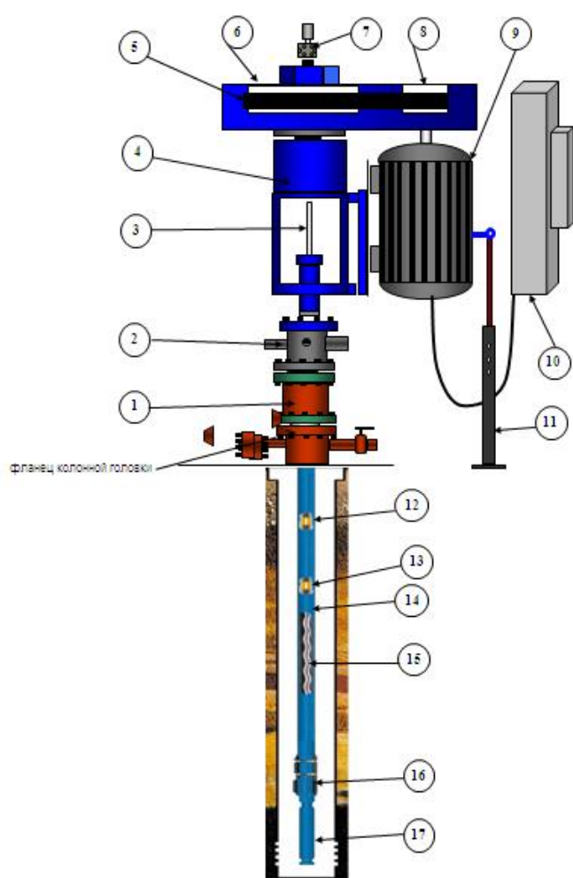
Рисунок 3. - Конструкция винтового насоса
