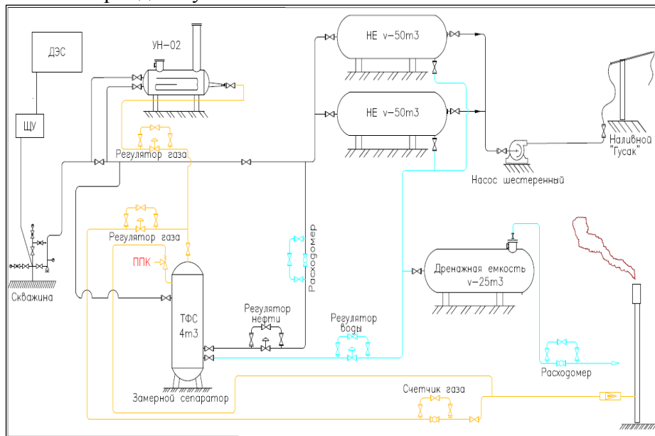
Рисунок 4 - Принципиальная индивидуальная технологическая схема сбора жидкости по скважине на период пробной эксплуатации месторождения Тайказан на период 01.01.2022 по 15.07.2023 гг.
