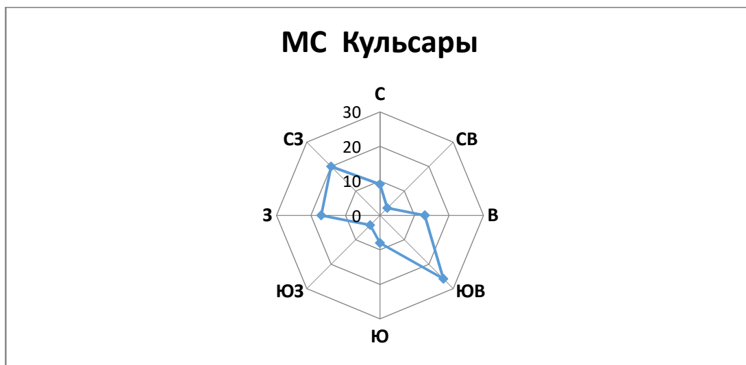
Рисунок 1.2.1- Роза ветров
