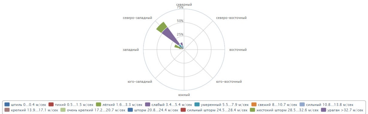
Рис. 7.2.1. Роза ветров
