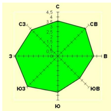
Рисунок 1.3 - Средняя годовая скорость ветра по румбам (%)
