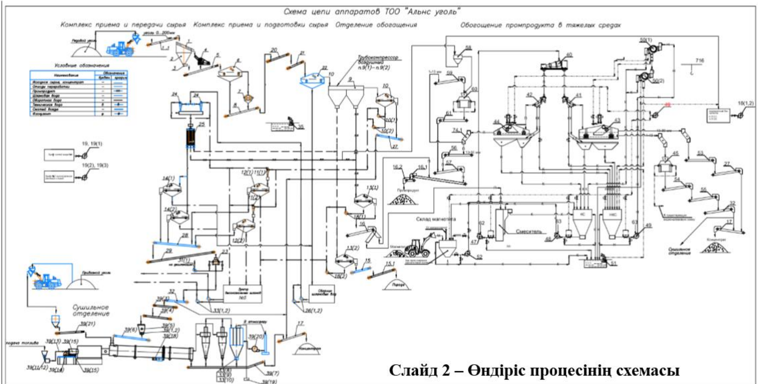
Слайд 2 – Схема производственного процесса
