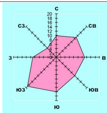
Рисунок 1.2 - Средняя годовая повторяемость направлений ветра и штилей (%)
