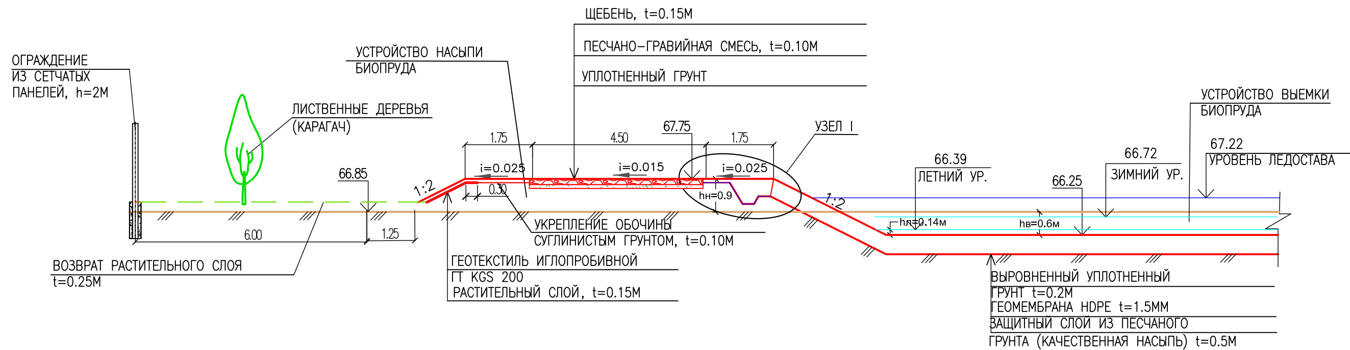
РАЗРЕЗ 1-1 М1:100
