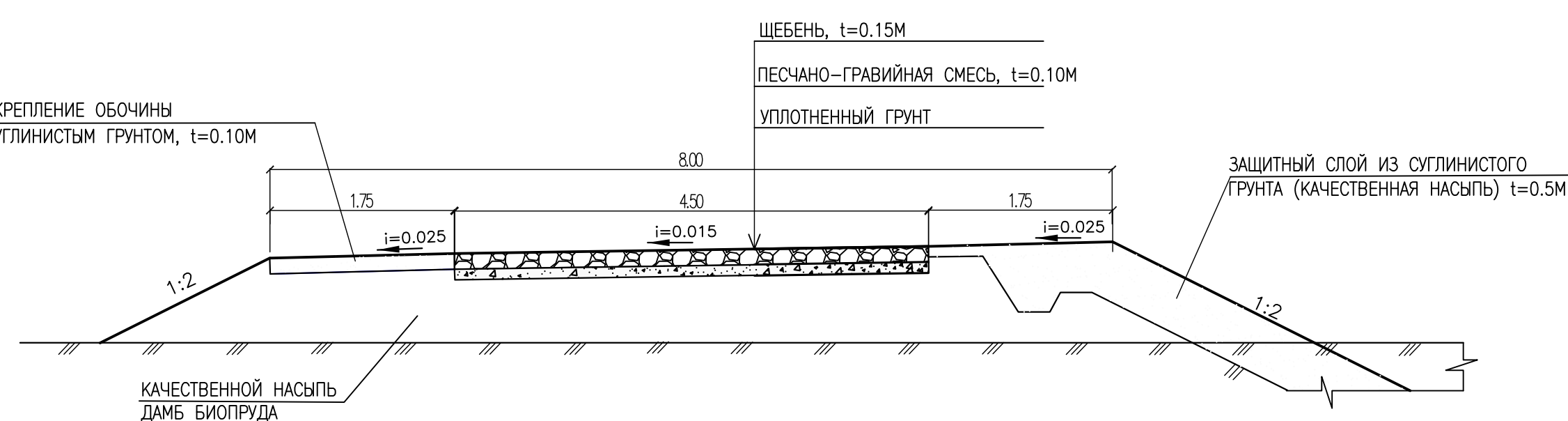
РАЗРЕЗ 3-3 М1:50 ПОКРЫТИЕ (ТИП 2)
