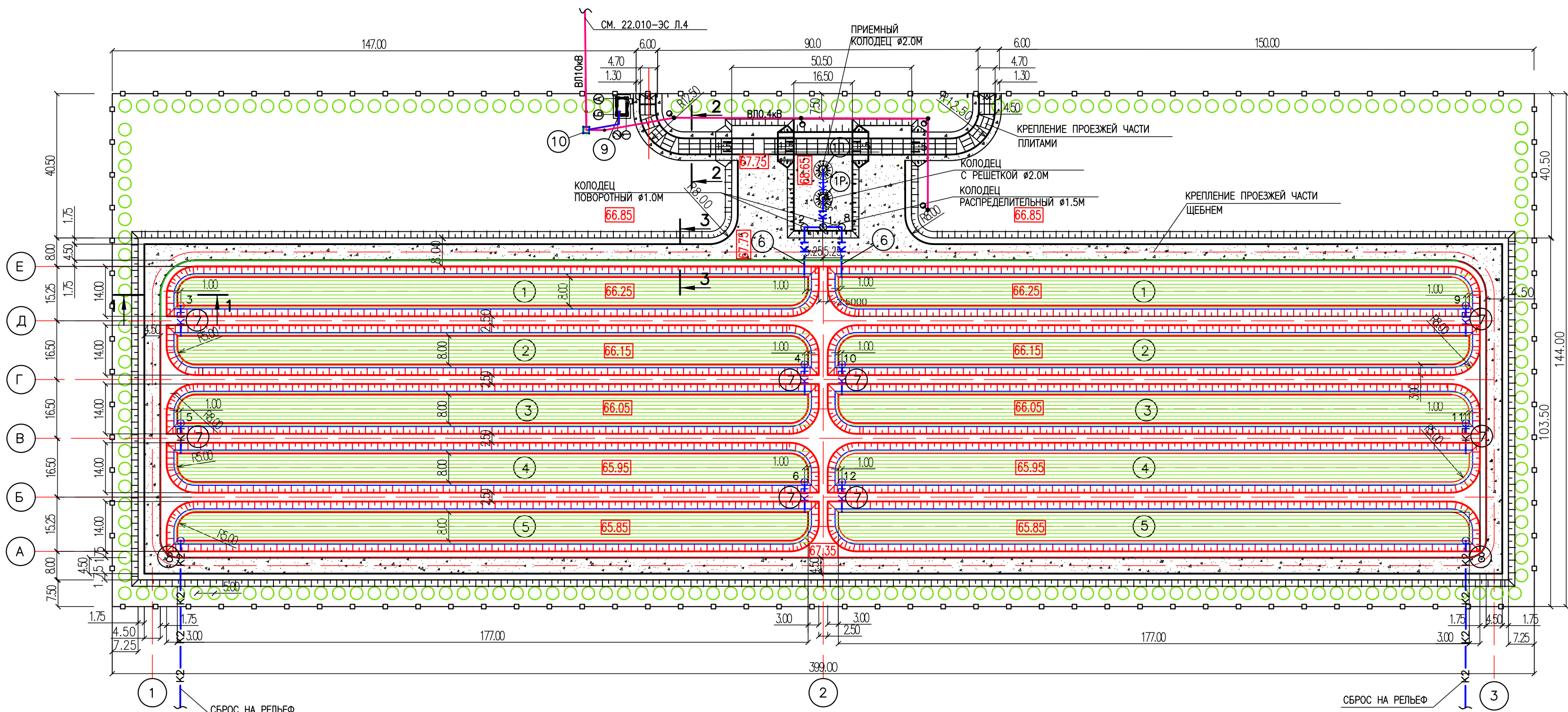
ПЛАН БИОПРУДА МАСШТАБ 1:1000
