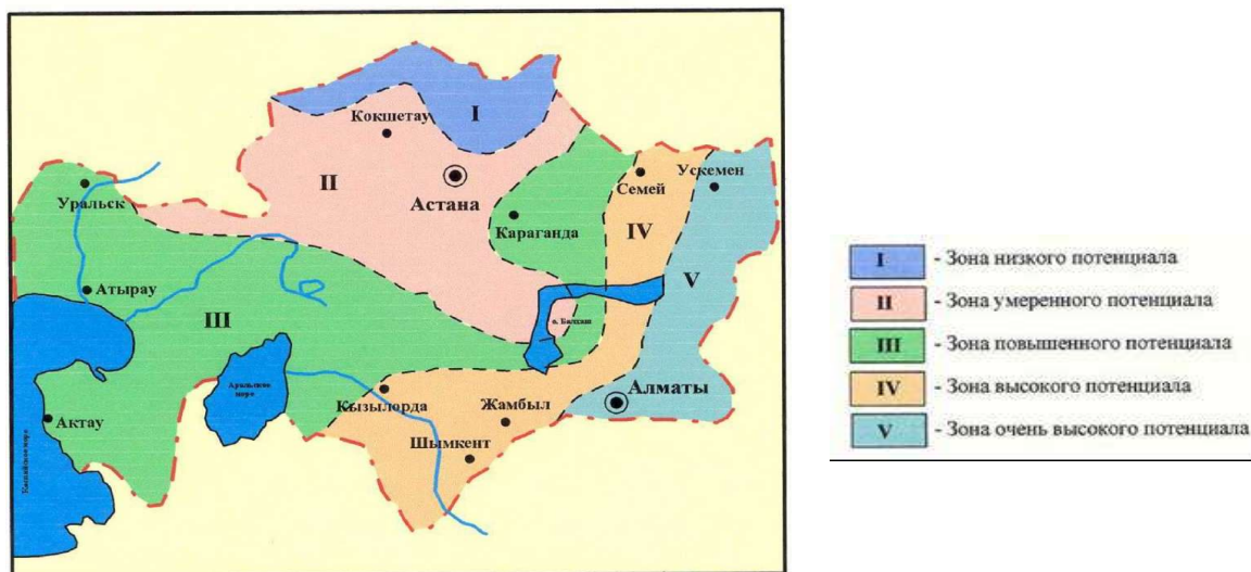
Рисунок 1.2.1.1 - Распределение значений потенциала загрязнения атмосферы для территории Республики Казахстан
