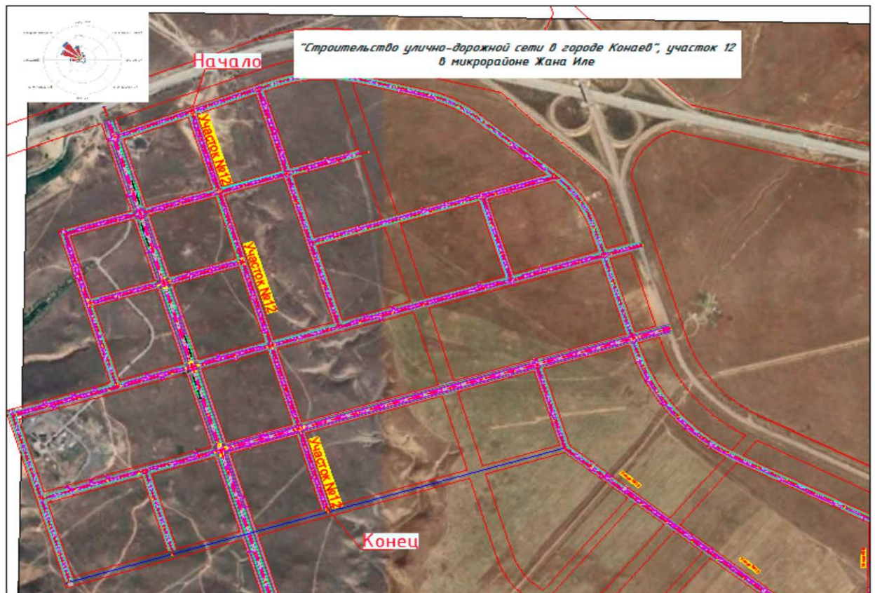
Рисунок 2.1 - Ситуационный план проектируемой улицы.
