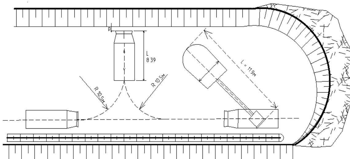
Рисунок 3.3 – Схема работы карьерной техники в зажатых условиях
