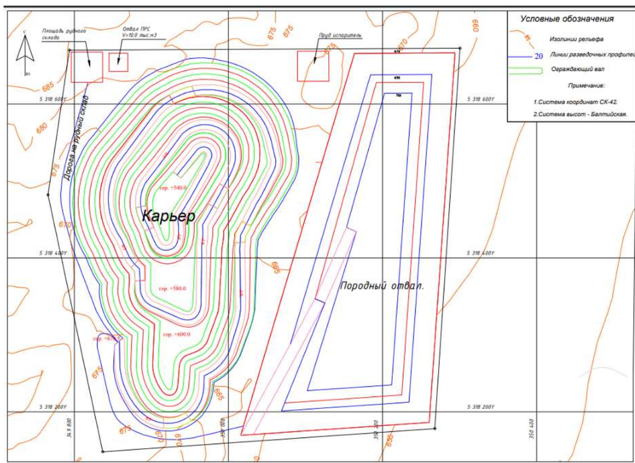
Рисунок 3.2 – Ситуационный план расположения объектов карьера
