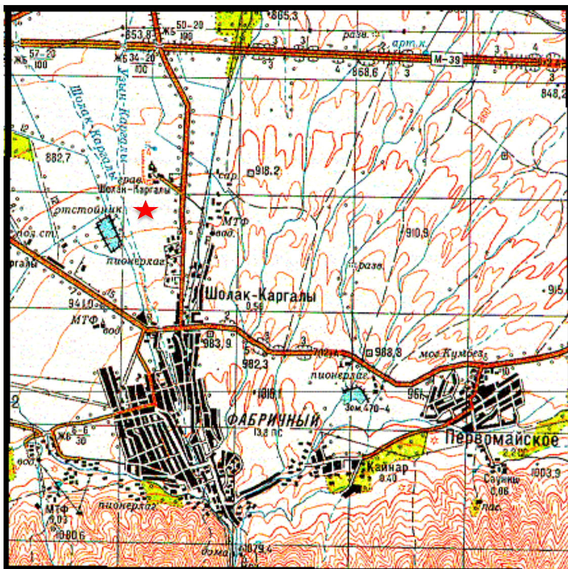
★ место рождения ПГС Шолпан-Каргалинское (Блок А-1) Рис 1.
