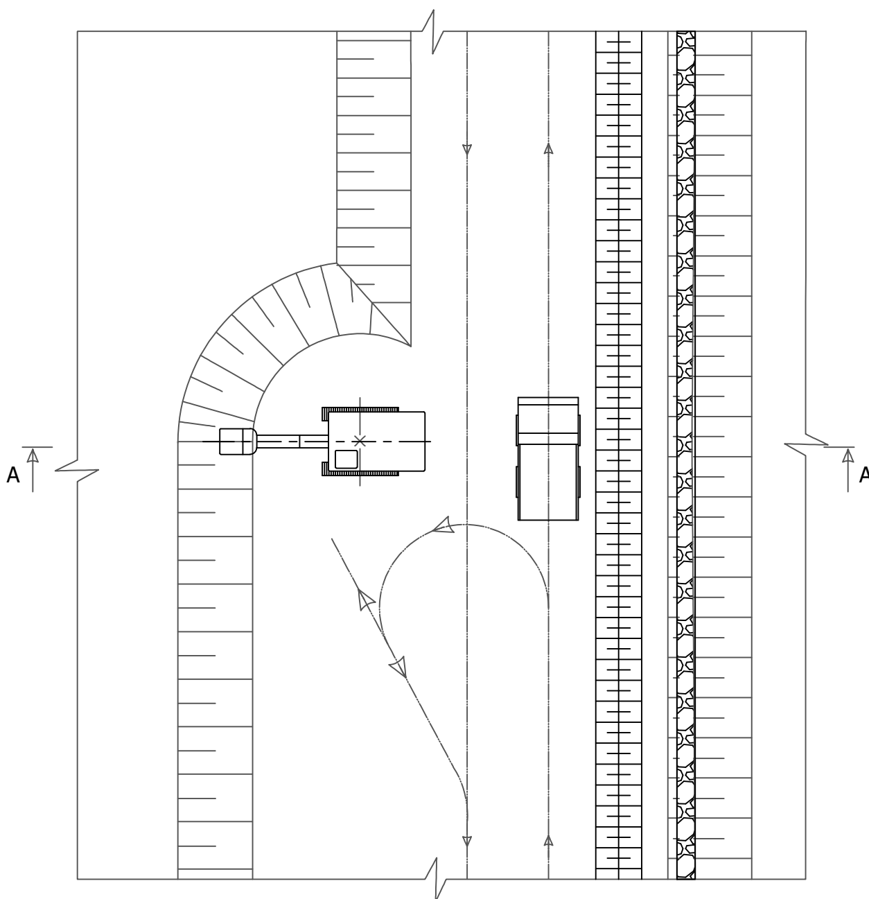
Технологическая схема отработки вскрышного уступа гидравлическим экскаватором (11м 3 ) с погрузкой в автосамосвалы 90т и 55т
