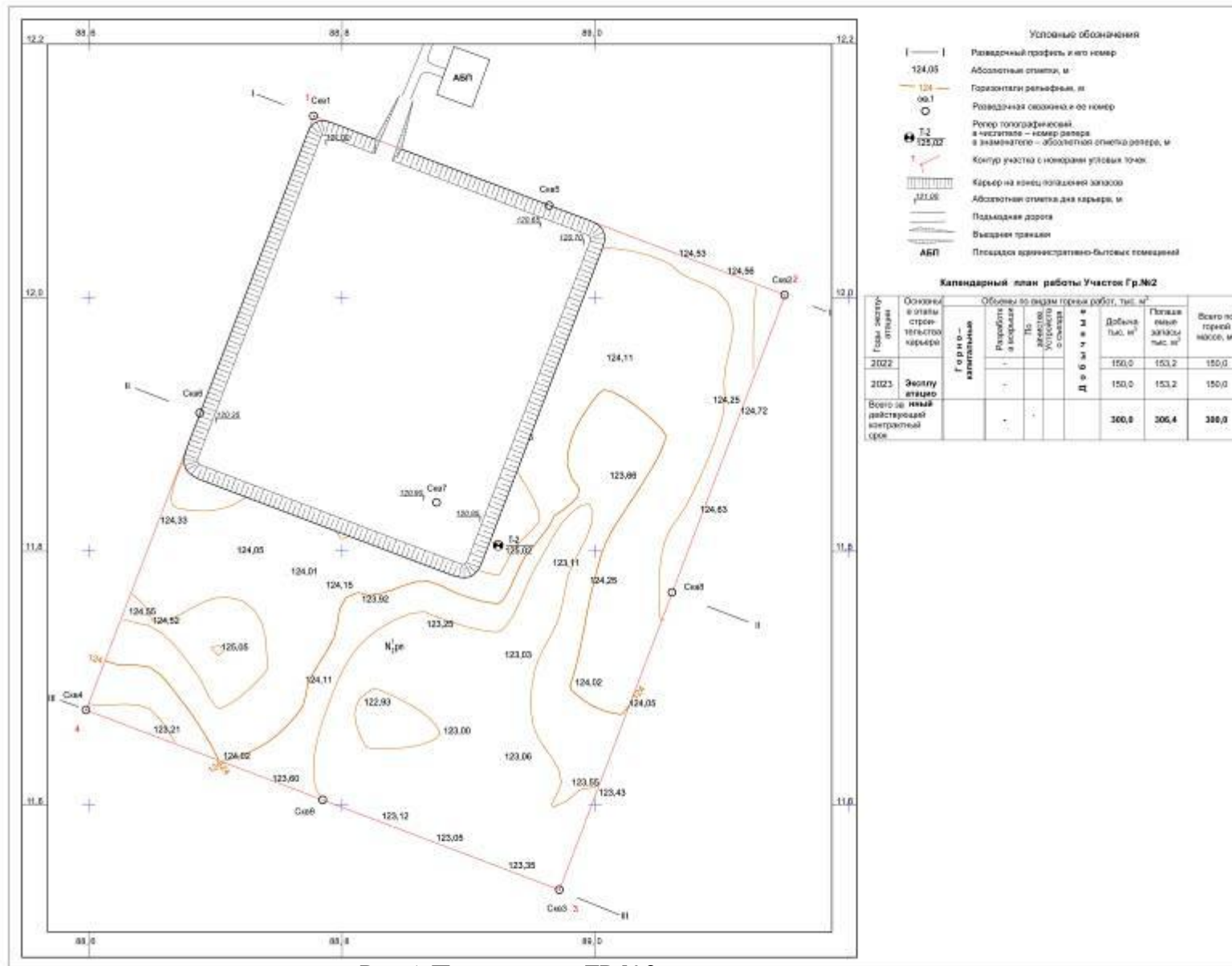
Рис.5. План карьера ГР №2 на конец погашения запасов
