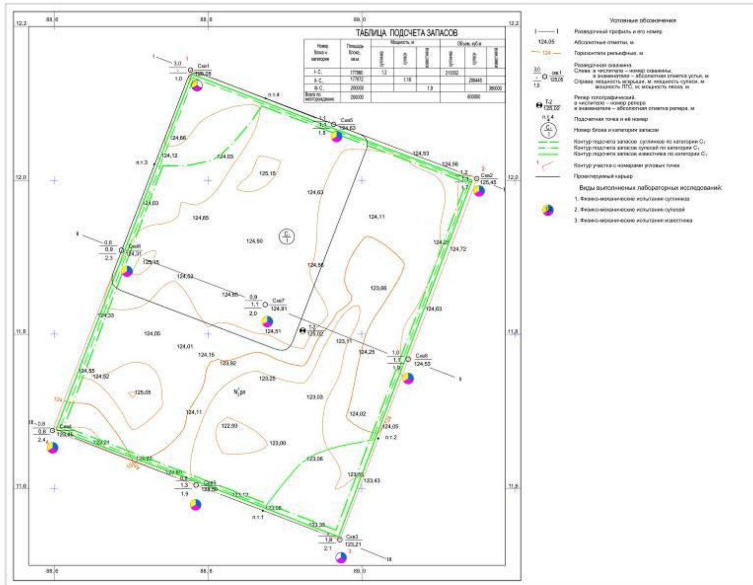
Рис.4. Топографический план местности проектируемого карьера ГР №2 на начало разработки
