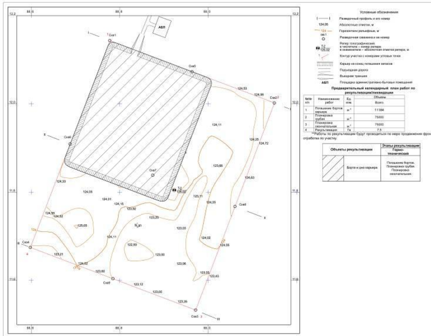
Рис.6. План проведения технической рекультивации нарушенных земель ГР №2
