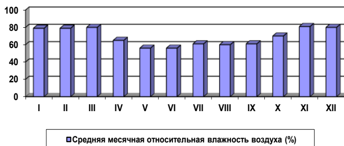
Рисунок 3.2 – Средняя месячная относительная влажность воздуха (%)
