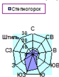
Рисунок 3.3 – Средняя годовая повторяемость направлений ветра и штилей (%)
