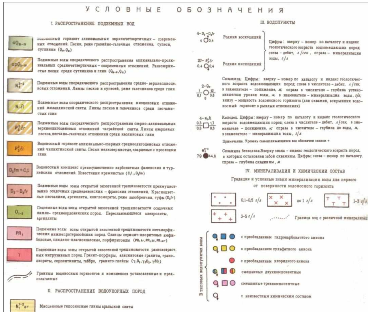
Рис.3. Условные обозначения к гидрогеологической карте района работ
