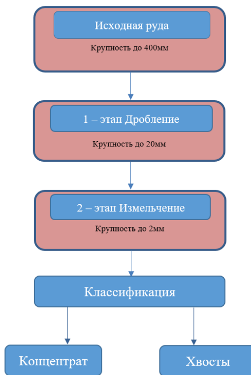
Рис. 4 – Технологическая схема
