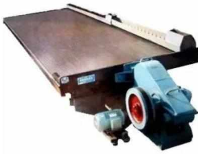
Рис. 5.7 – Стол концентриционный
