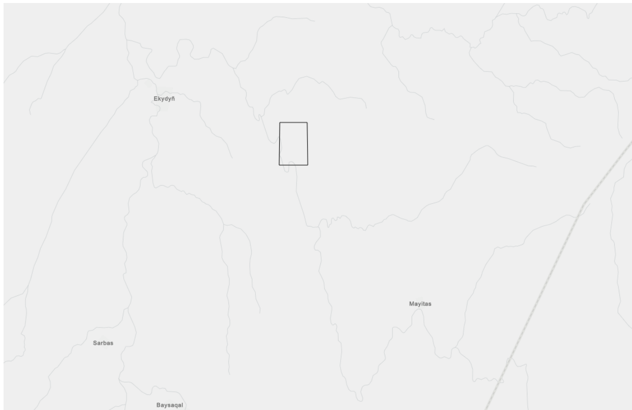
Рисунок 1.2 Картограмма расположения лицензионной территории участка Караторгай
