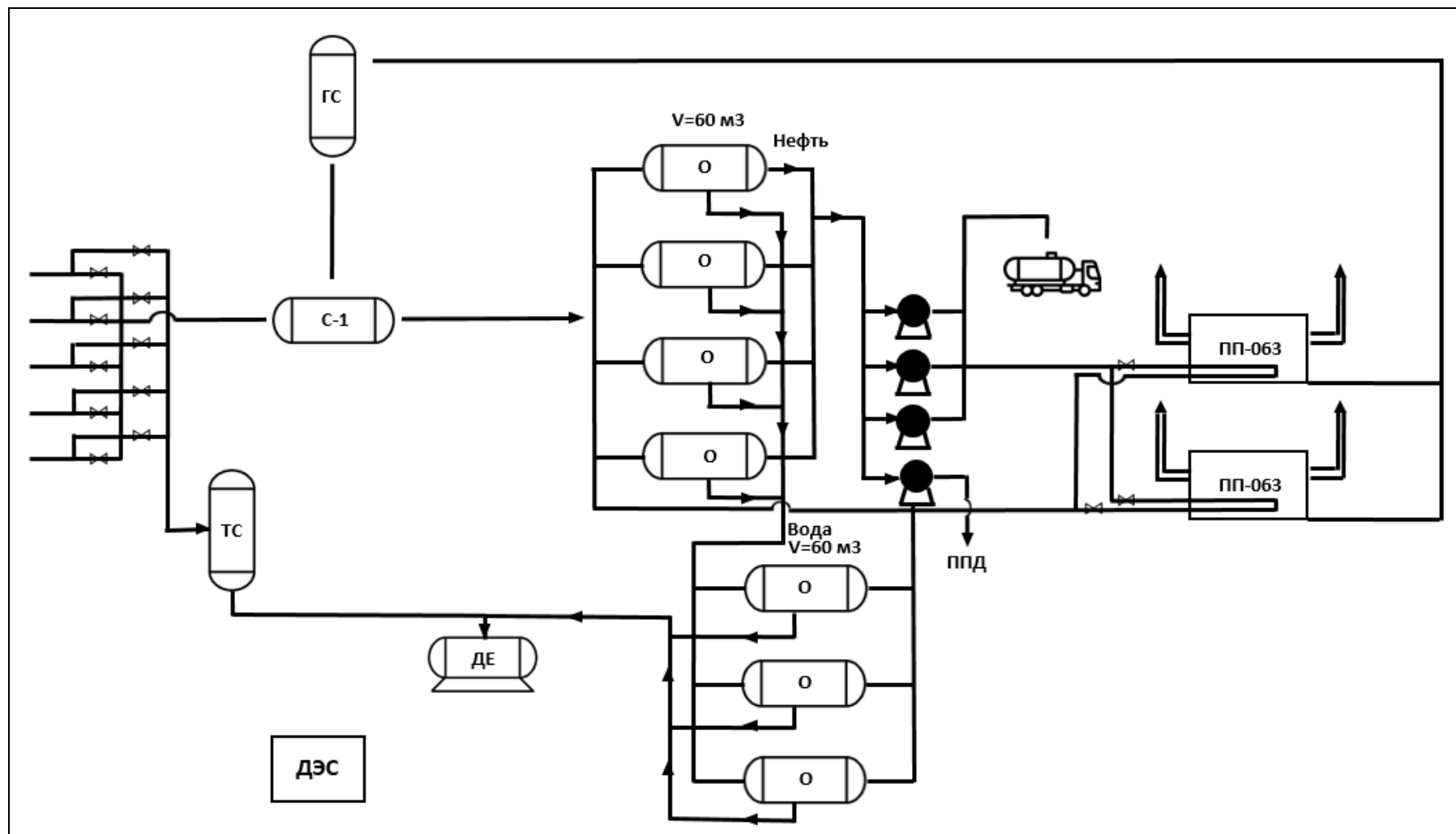
Рис.3– Существующая система сбора подготовки нефти на месторождении месторождения Кумысбек
