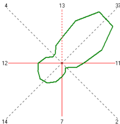
Рис 3 - Роза ветров
