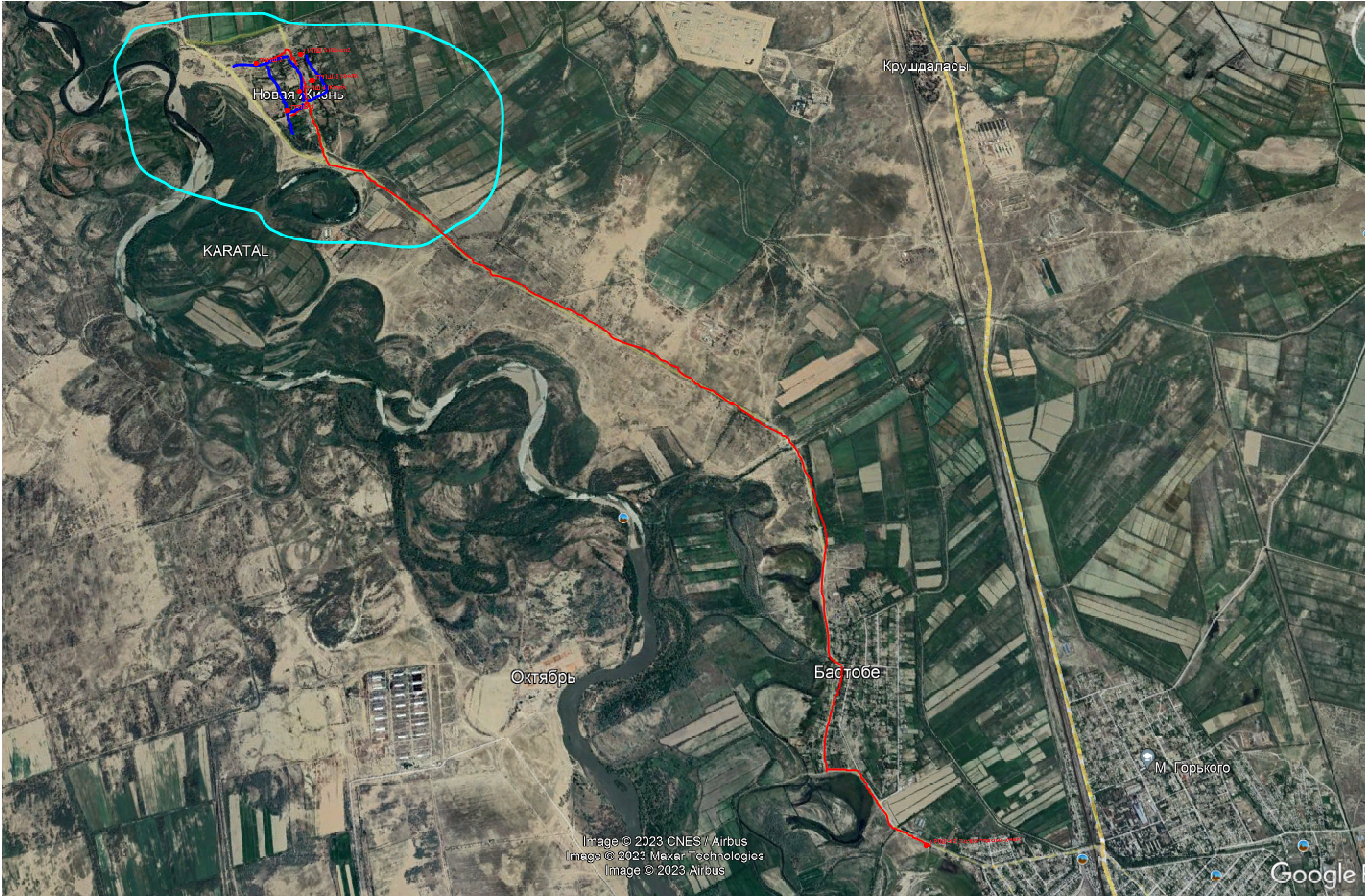
Ситуационная схема подводящего газопровода и газораспределительных сетей с. Кишитобе, Каратальского района области Жетісу
