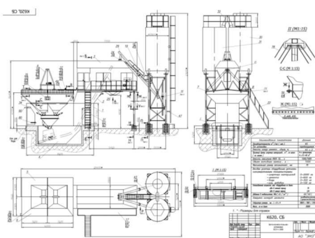
Принцип работы БСУ-1000:
