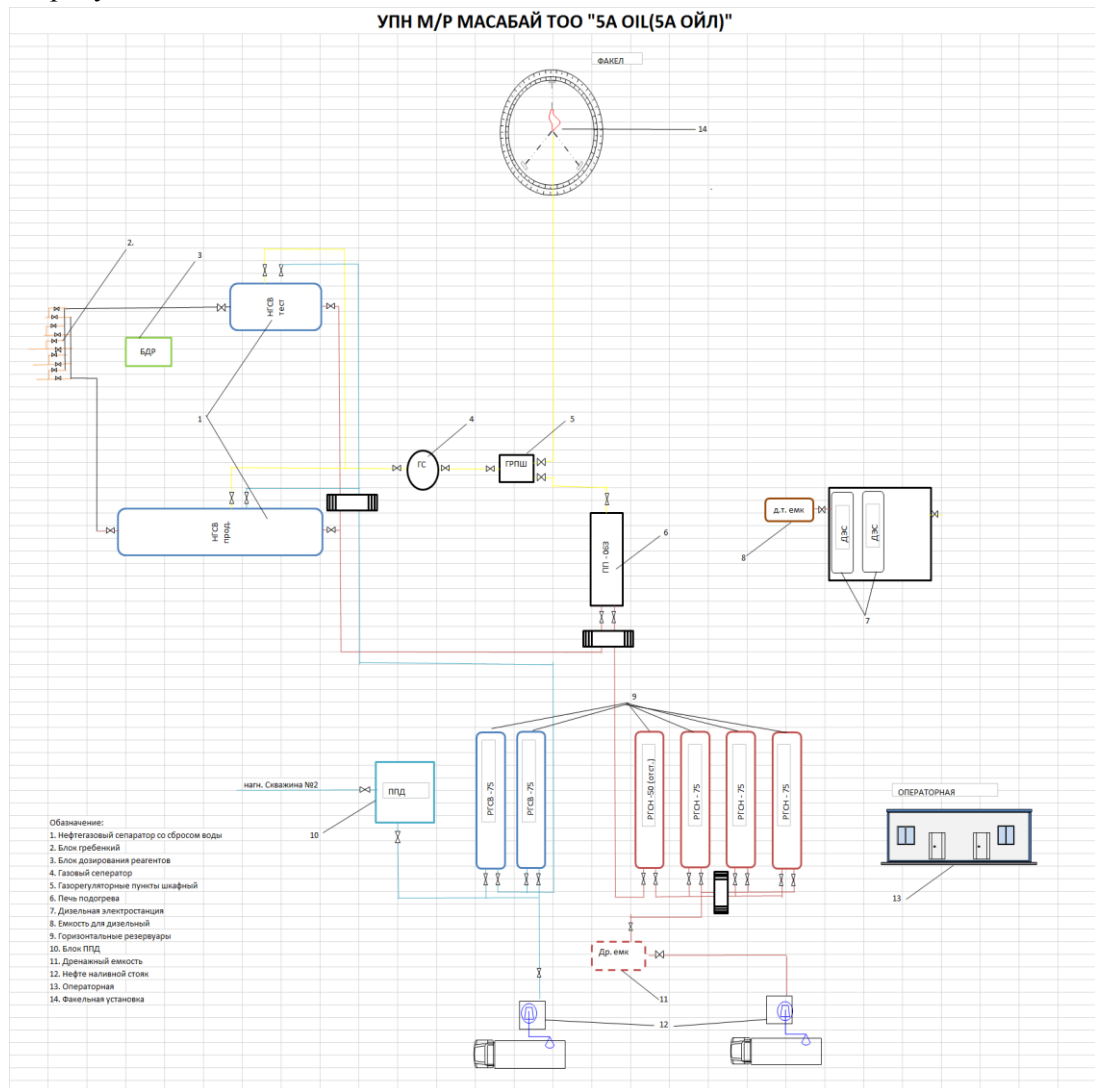
Рисунок 8. Существующая схема системы сбора и подготовки нефти месторождения Масабай
