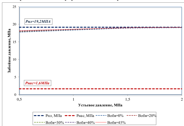
Рисунок 7. Объект-III. Зависимость минимальных забойных давлений фонтанирования от давления на устье (НКТ=73 мм)
