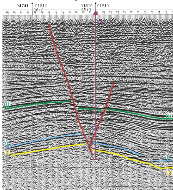
Рис.5 - Фрагмент временного разреза 018103
