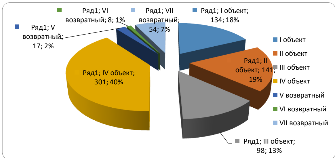
Рисунок 5– Распределение геологических запасов нефти по объектам
