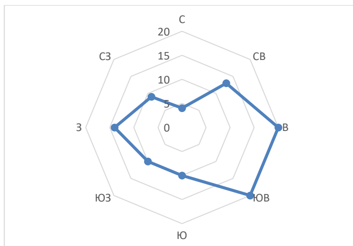
Рис. 9.1.1.1 – Роза ветров
