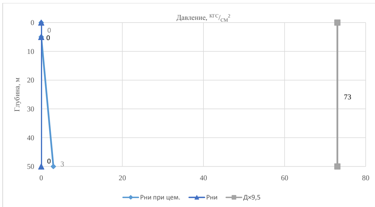
Рисунок 9.1 – Эпюра избыточных наружных давлений, действующих на направление Ø323,9 мм
