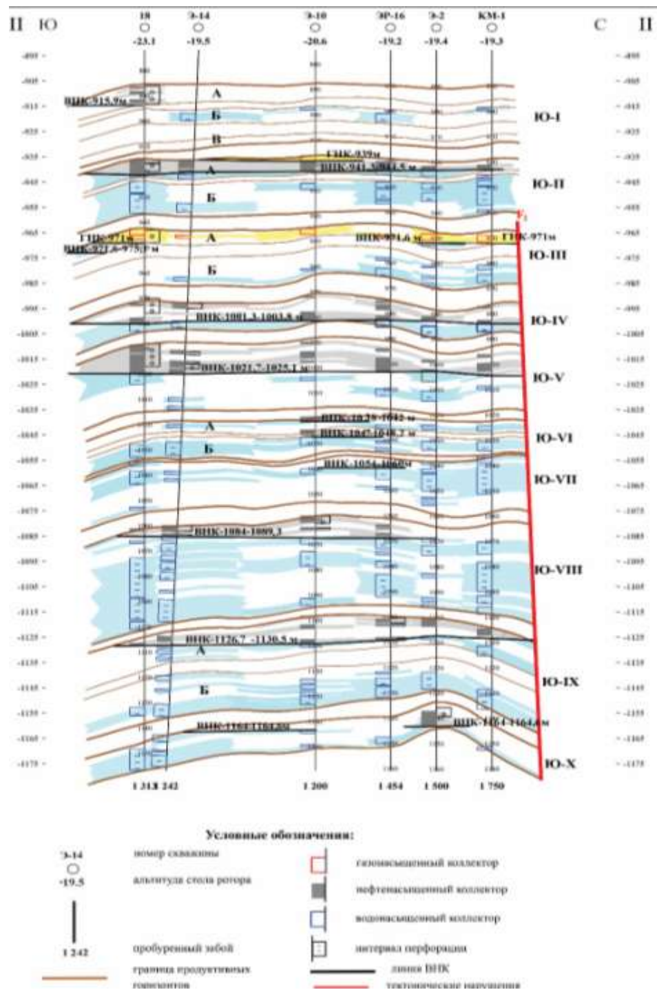
Рисунок 4.6 – Каратурун Морской. Геолого-литологический профиль
