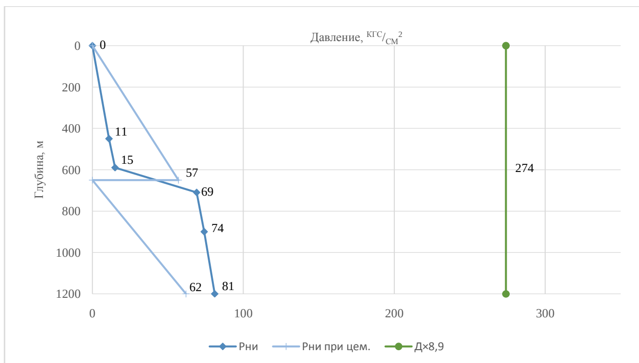
Рисунок 9.5 – Эпюра избыточных наружных давлений, действующих на эксплуатационную колонну Ø 168,3 мм
