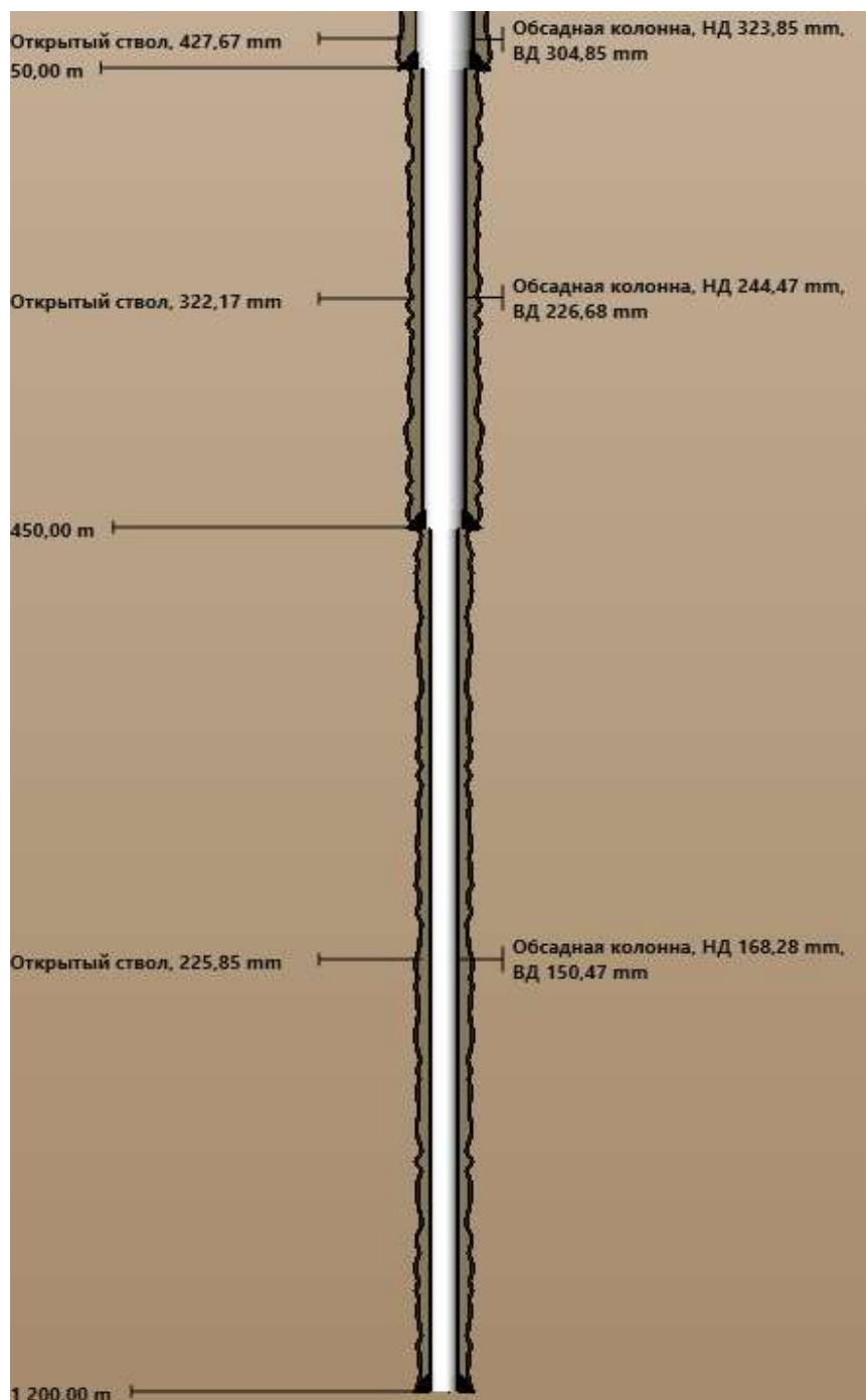
Рисунок 6.1– Проектный профиль скважины
