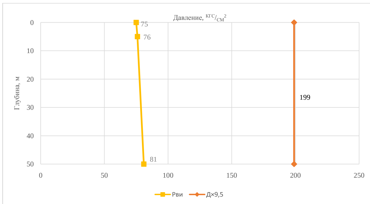
Рисунок 9.2 – Эпюра избыточных внутренних давлений, действующих на направление Ø 323,9 мм
