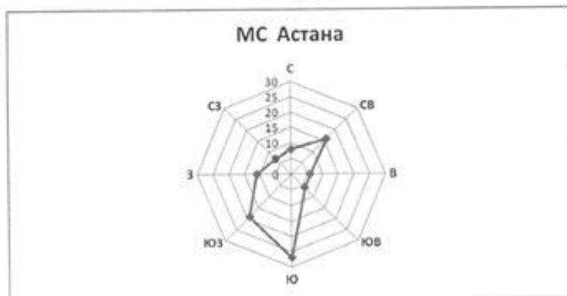
Роза ветров
