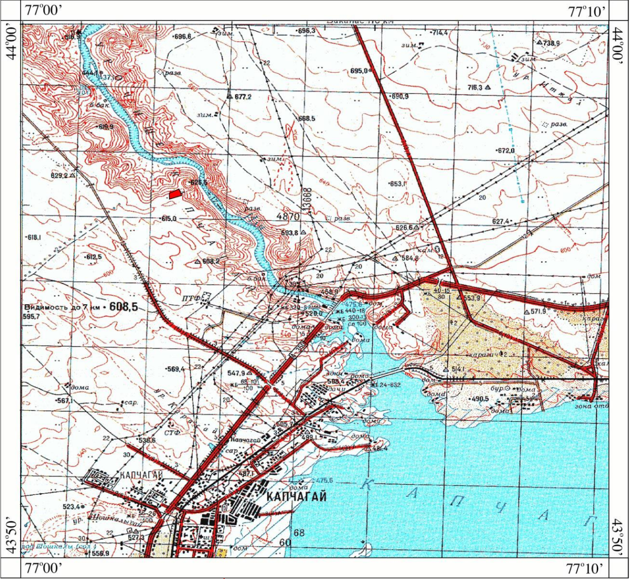
Участок Капчагайское-8 Рис.1 Обзорная карта расположения месторождения
