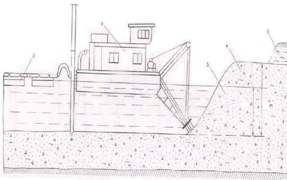
Принципиальная схема разработки уступа плавучим земснарядом. 1- земснаряд; 2-плавучий пульповод; 3-подводная часть уступа; 4-надводная часть уступа; 5 почвенный слой.
