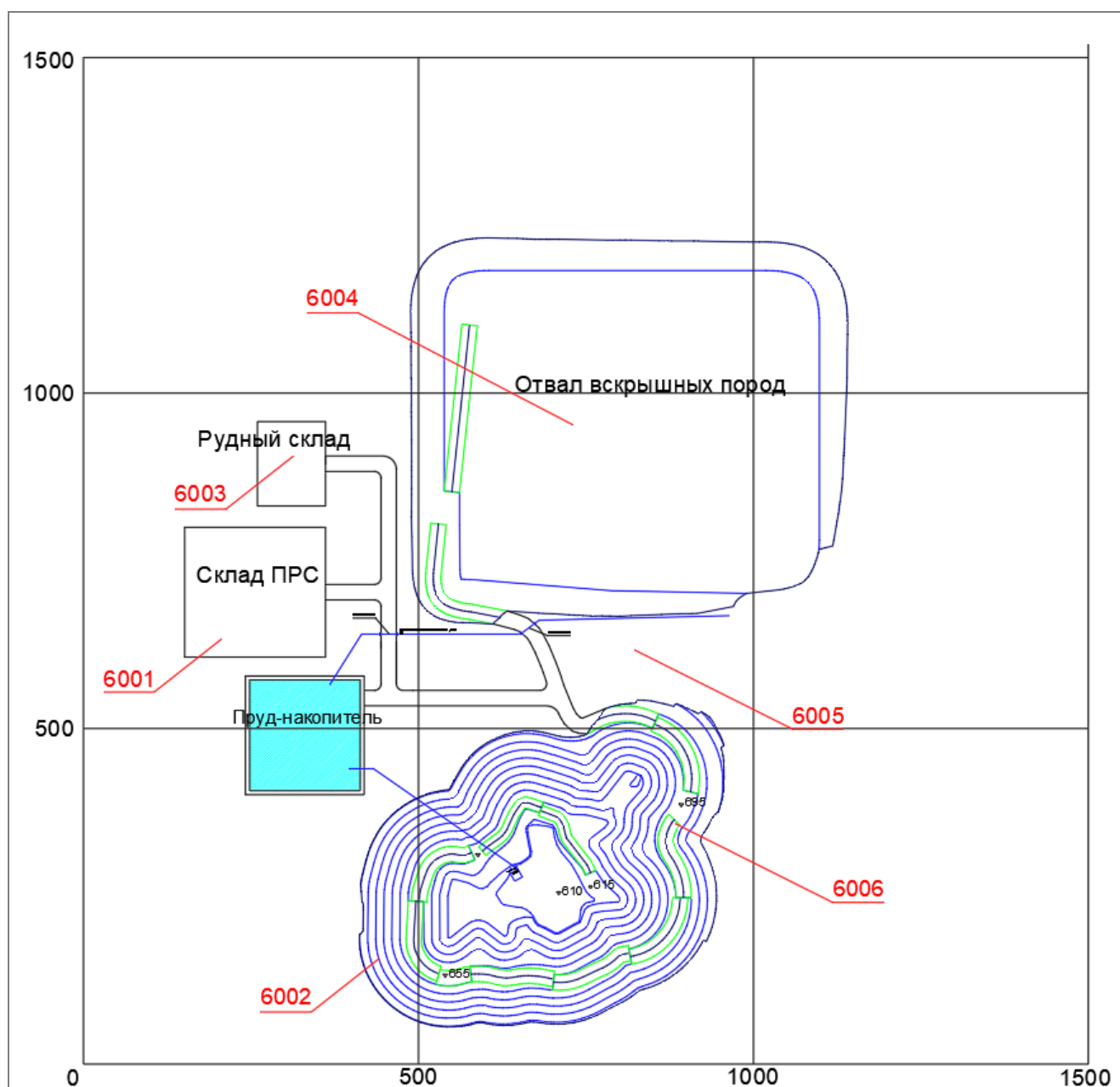
Рисунок 7 Размещение источников выбросов на площадке предприятия
