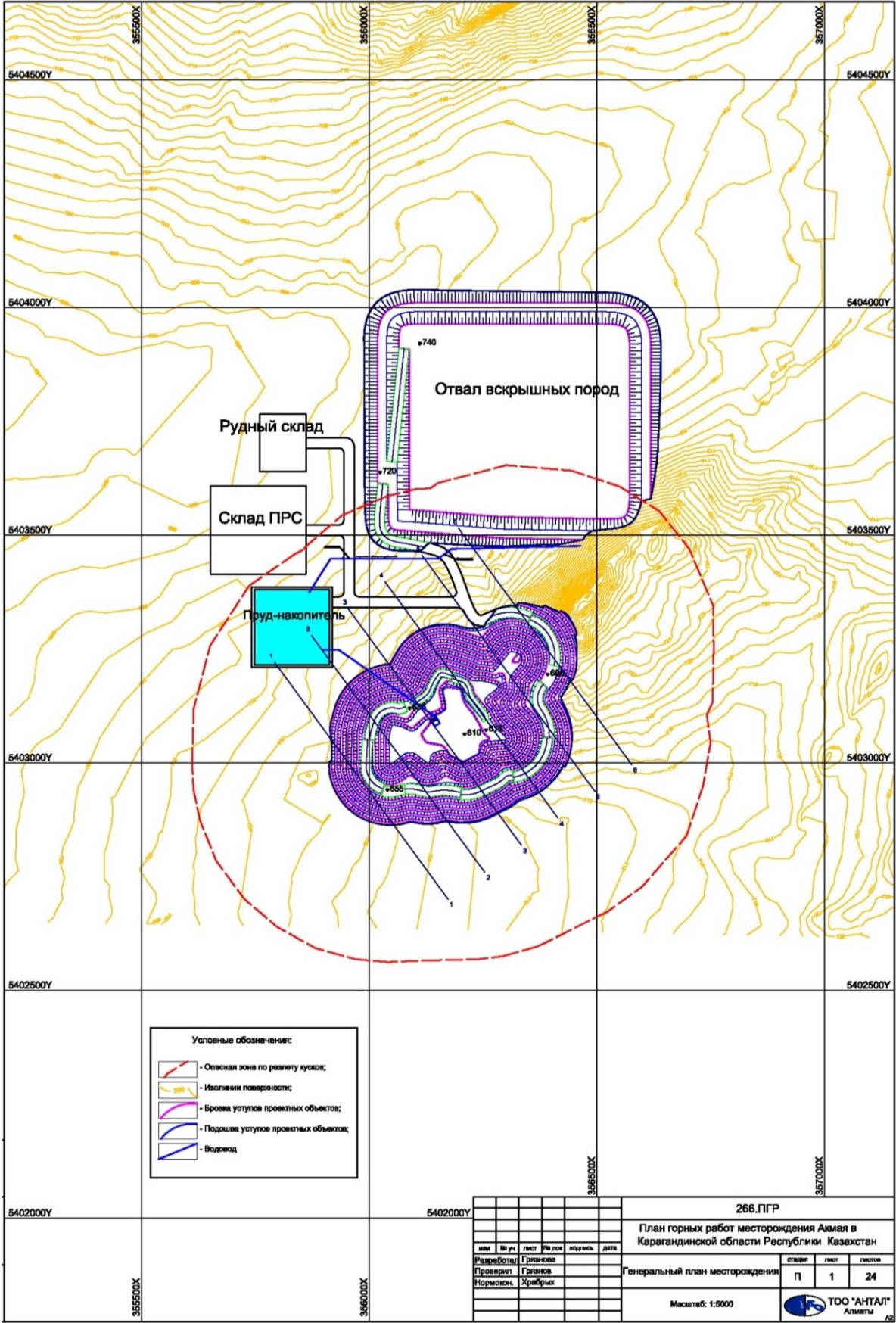
Рисунок 6 Генеральный план месторождения Акмая
