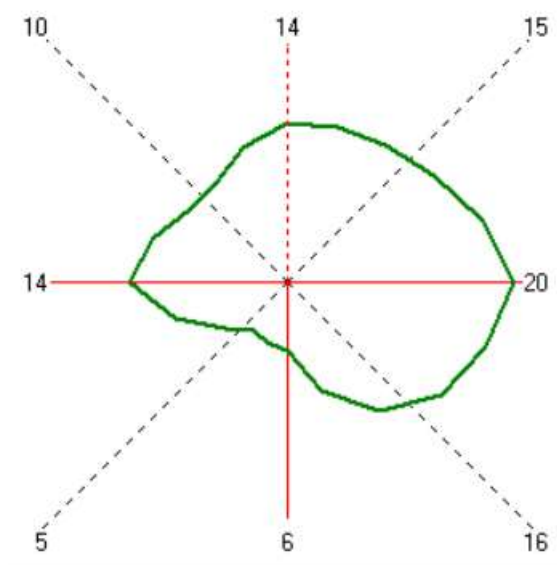
Рис 2 - Роза ветров
