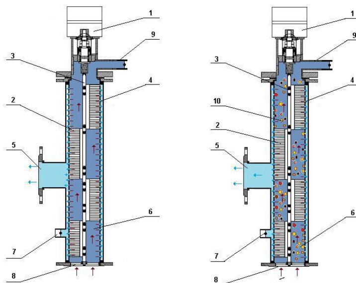
Рисунок 16.2 – Процесс очистки в фильтрах ССФ (1 – электропривод; 2 – щетка; 3 – ось; 4 – внутренняя поверхности сетки; 5 – фланец патрубка вывода очищенной жидкости; 6 – исходная жидкость; 7 – патрубок обратной промывки;
