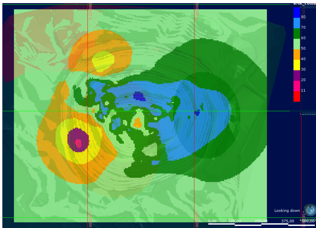
Рисунок 2.2 - Блочная модель месторождения Пустынное качества массива по рейтингу BRMR (Бенявского).
