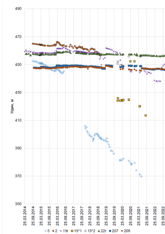
Рисунок 1.7 - Графики изменения динамического уровня воды в наблюдательных скважинах № 005GT, 002GT, 19г, 22г, 207сн и 208сн, расположенных в пределах возможной области дренирующего влияния карьера.
