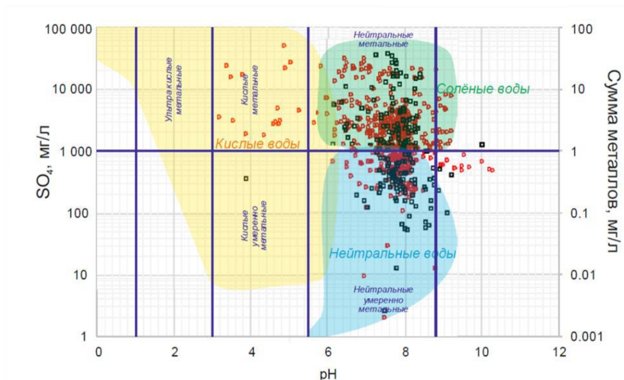
Рисунок 1.10 – Диаграмма У. Фиклина типов вод в пределах объекта исследований по зависимости концентрации сульфатов и суммы металлов от pH.
