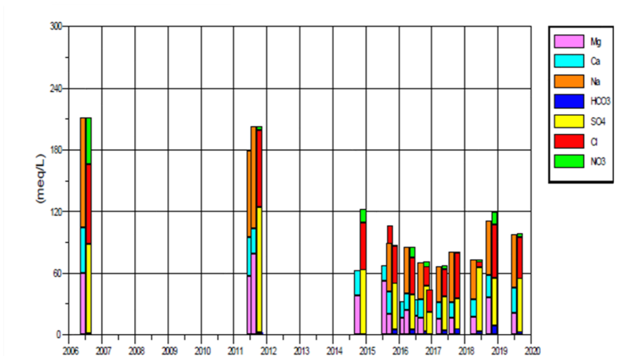
Рисунок 1.8 -График изменения катионного и анионного состава карьерных вод месторождения Пустынное.
