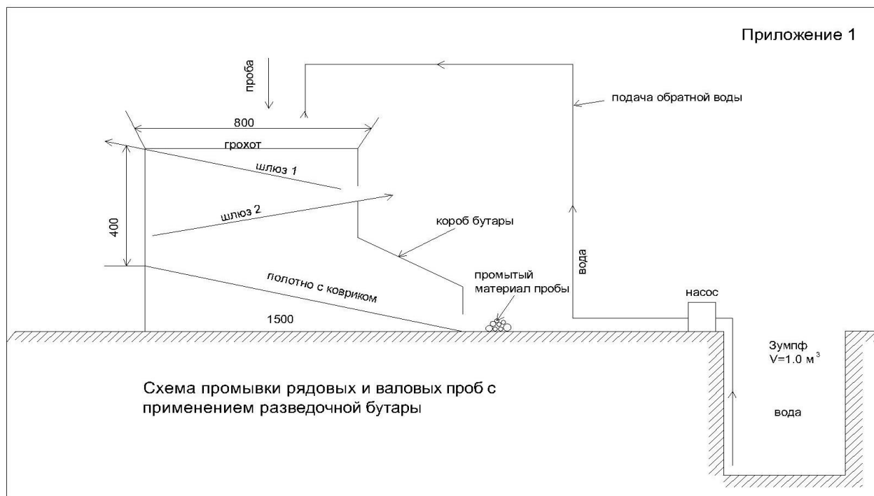
Рис. 2.3.1 Схема промывки рядовых и валовых проб с применением разведочной бутары
