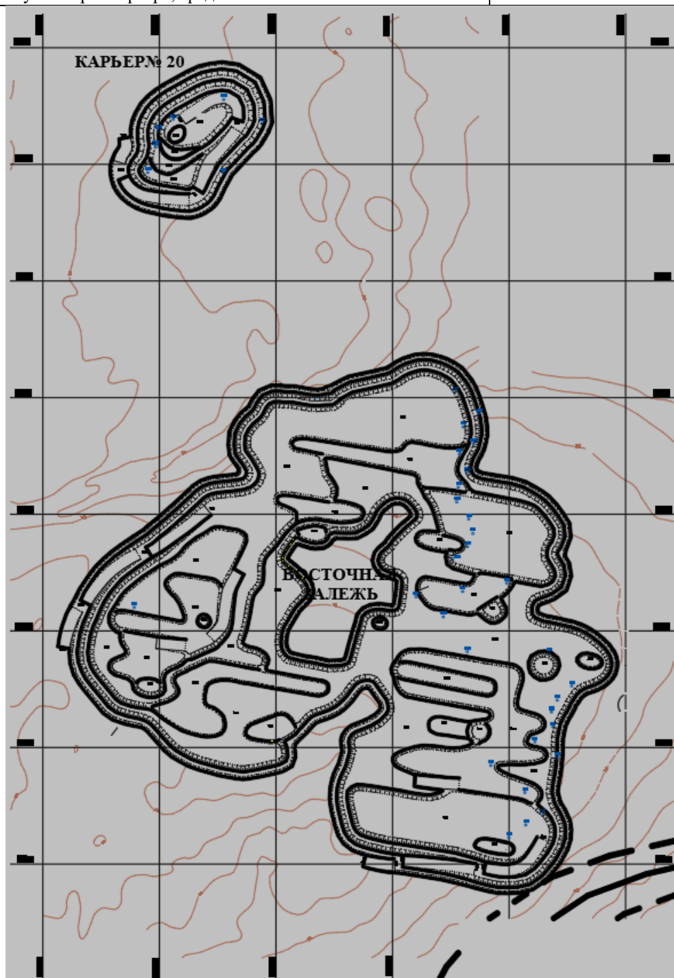
Рисунок 3.1 – План карьера 20 и карьера Восточной залежи на конец отработки
