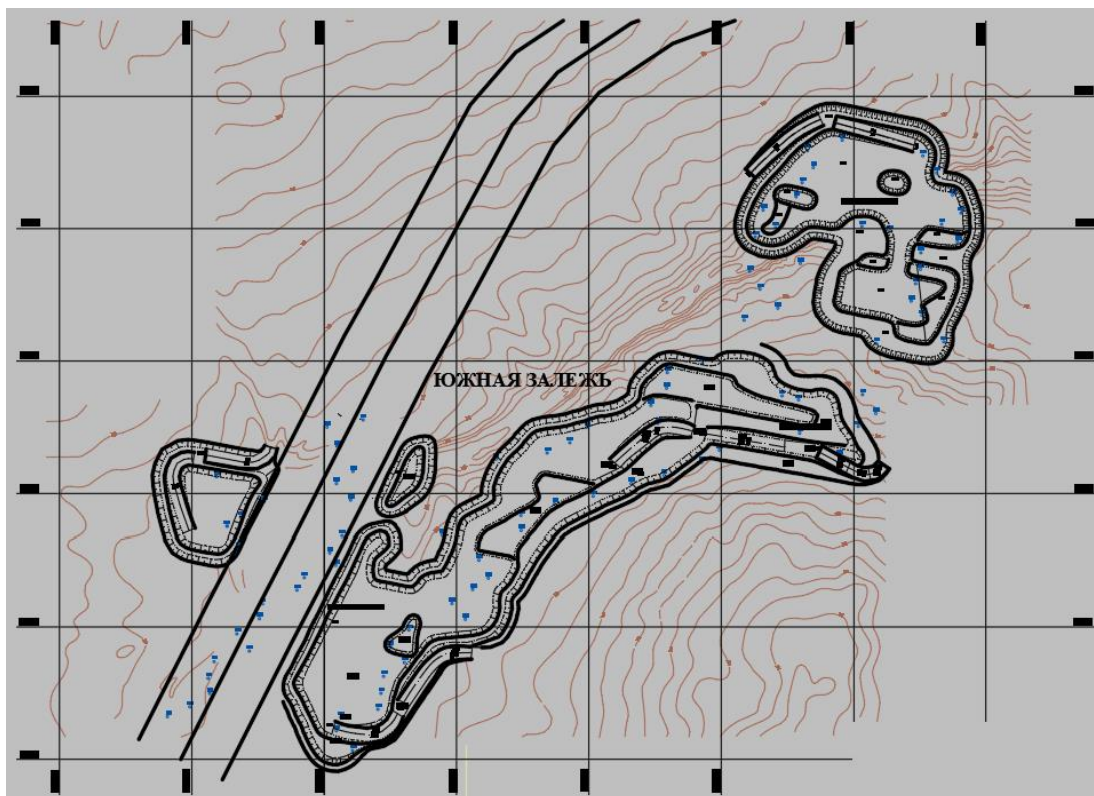
Рисунок 3.2 – План карьера Южной залежи на конец отработки
