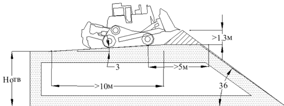
Рисунок 4.3.- Формирование разгрузочной площадки отвала бульдозером
