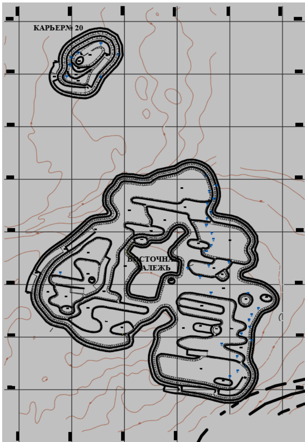
Рисунок 3.1 – План карьера на конец отработки
