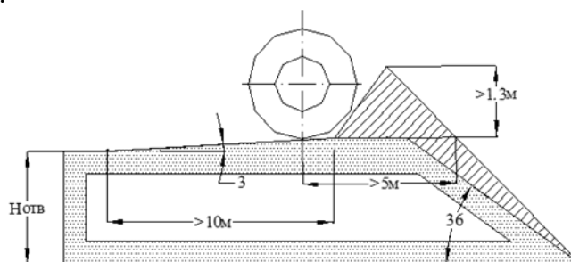
Рисунок 4.2. - Схема разгрузочной площадки отвала
