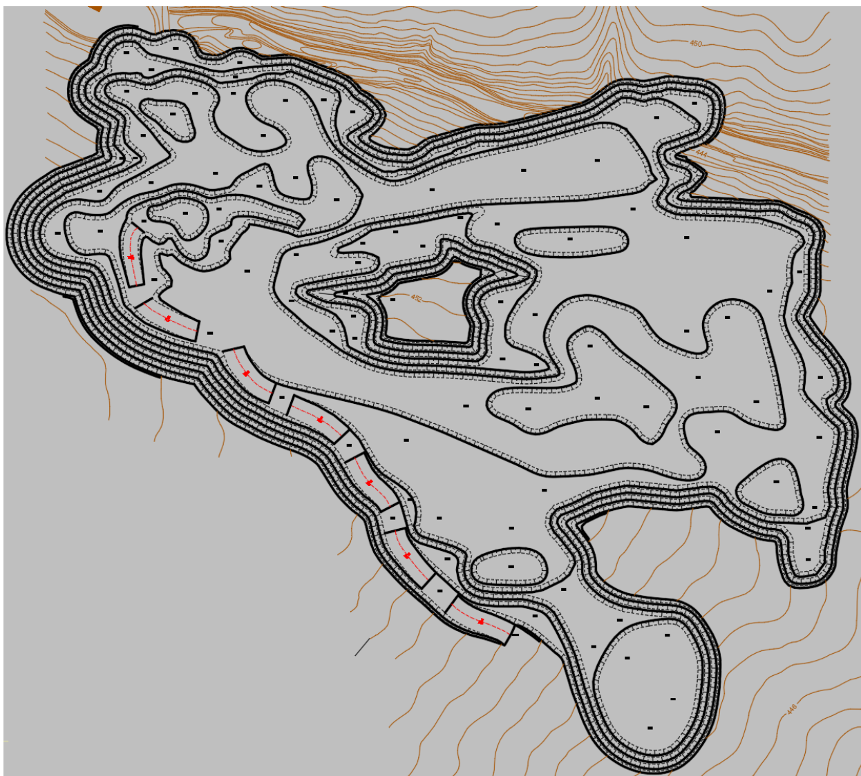
Рисунок 3.1 – План карьера на конец отработки
