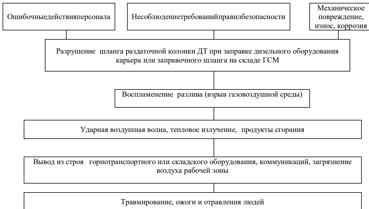
Рисунок 10.2 - Блок-схема вероятного сценария возникновения и развития аварии при заправке дизельного технологического оборудования карьера из топливозаправщика или заправке емкости на складе ГСМ
