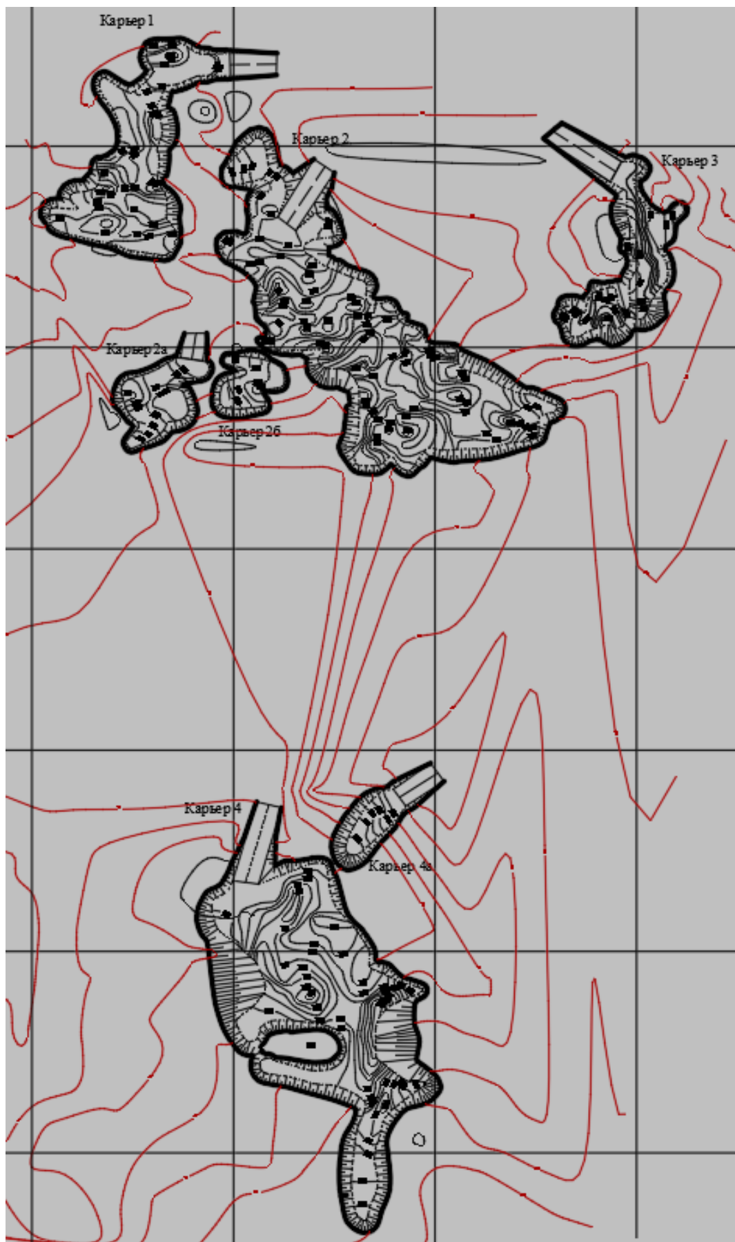
Рисунок 3.1 – План карьера на конец отработки
