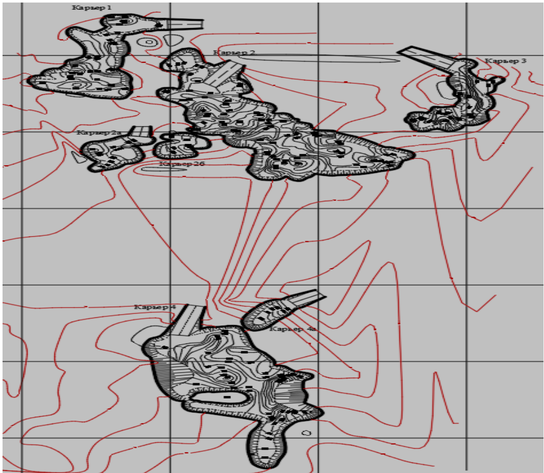
Рисунок 3.1 – План карьера на конец отработки
