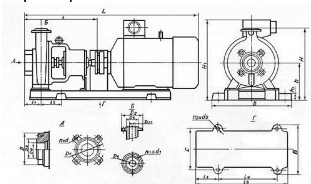
Габаритныйчертеж
