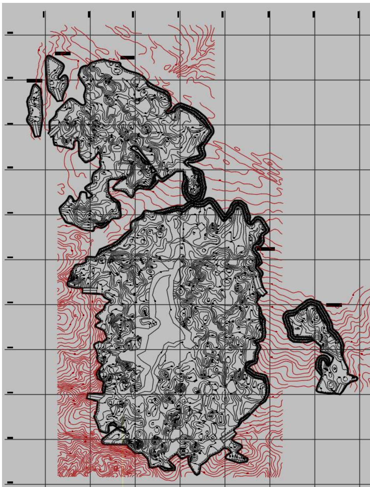
Рисунок 3.1 – План карьера на конец отработки
