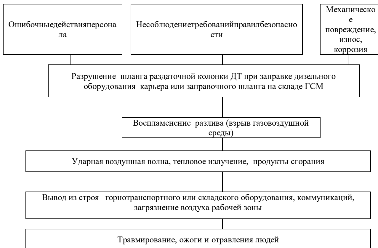
Рисунок 10.2 - Блок-схема вероятного сценария возникновения и развития аварии при заправке дизельного технологического оборудования карьера из топливозаправщика или заправке емкости на складе ГСМ
