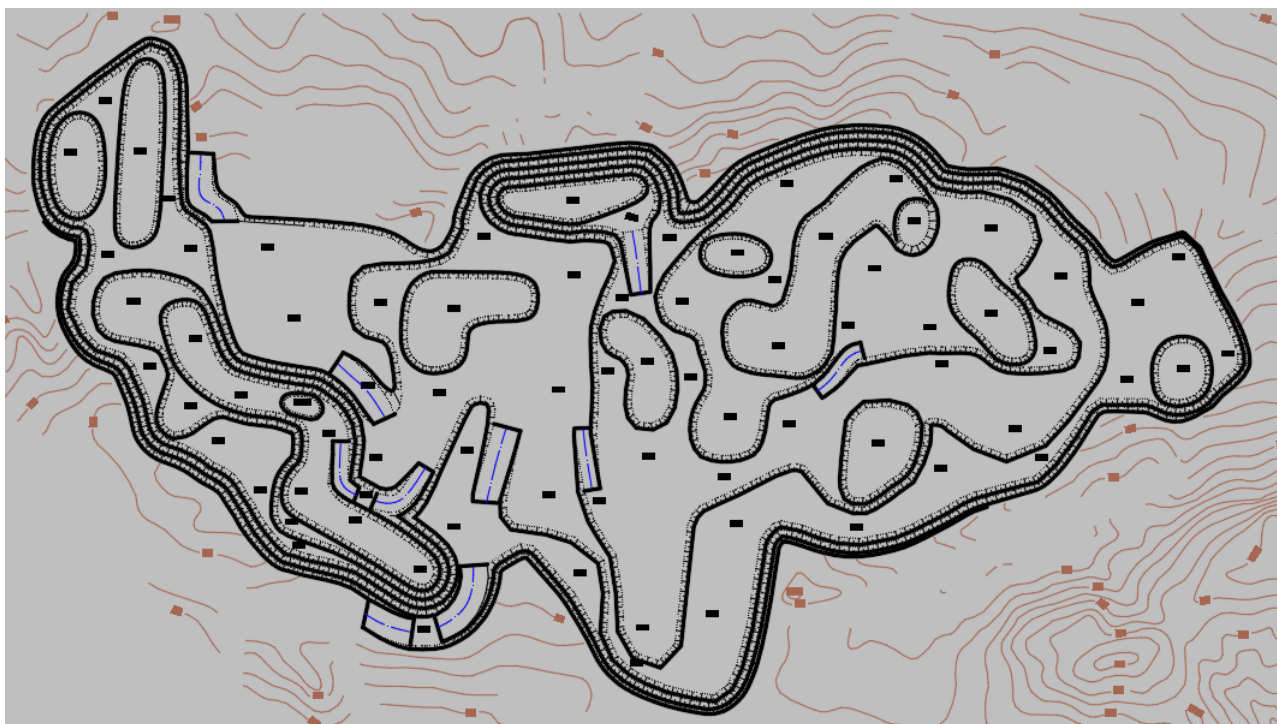
Рисунок 3.1 – План карьера на конец отработки
