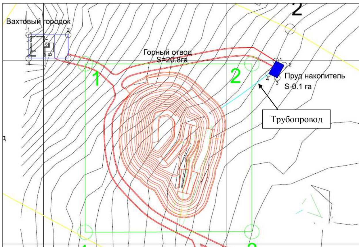
Рисунок 1.6 План расположения трубопровода с карьера месторождения Коскудук в пруд-накопитель
