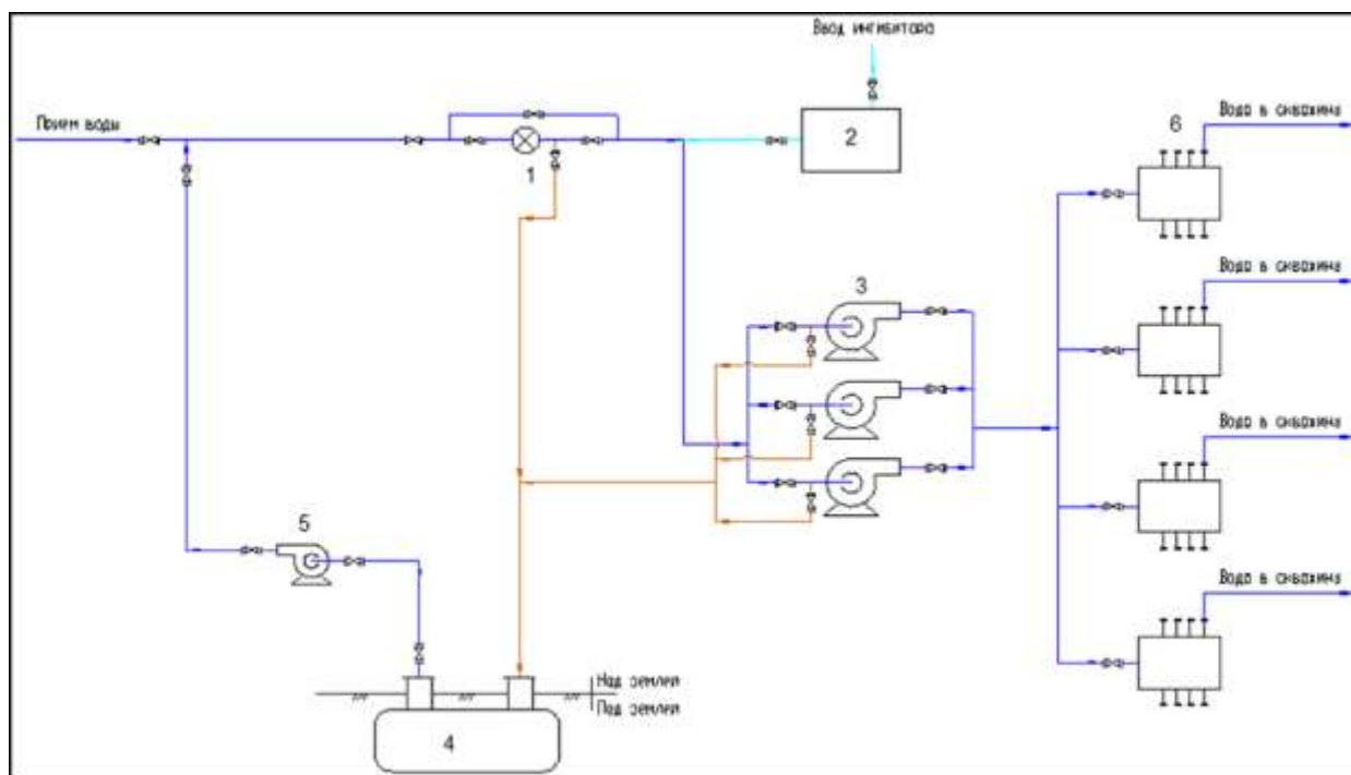
Рисунок 4.2 –принципиальная технологическая схема бкнс
