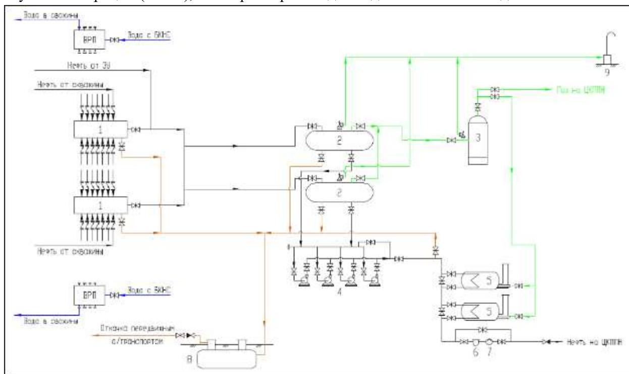
Рисунок 4.1 – Принципиальная схема ГУ на месторождении Каламкас
